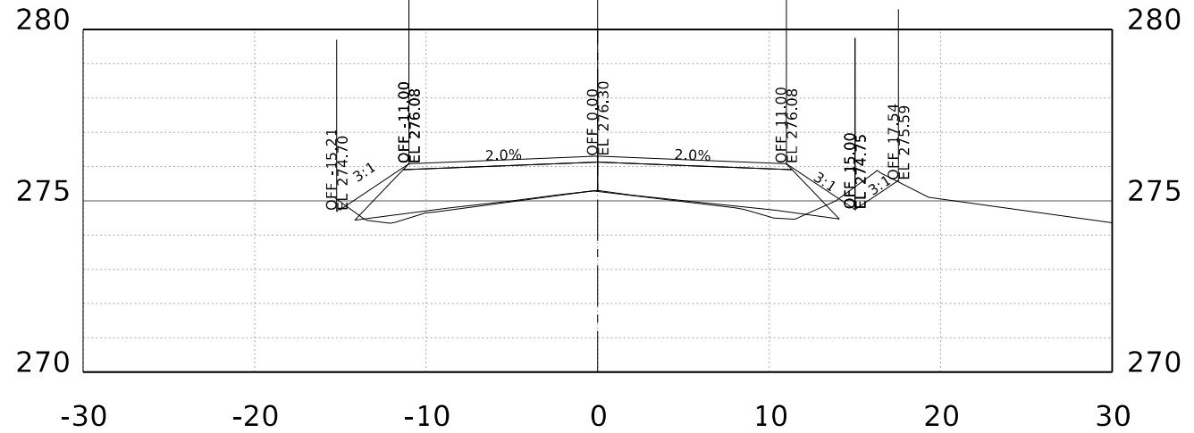
STA. 137+00.00 R1
