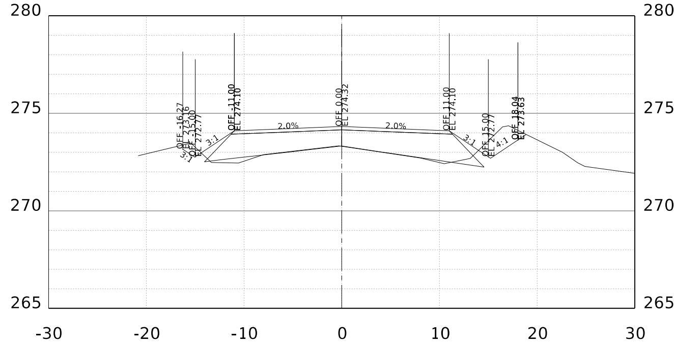
STA. 139+00.00 R1
