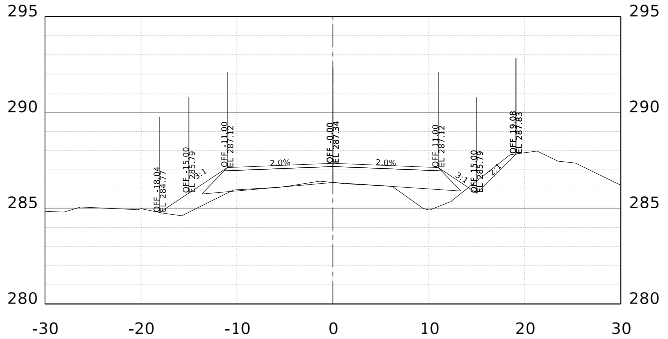
STA. 122+00.00 R1
