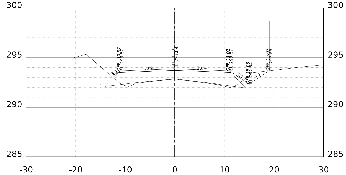
STA. 126+00.00 R1
