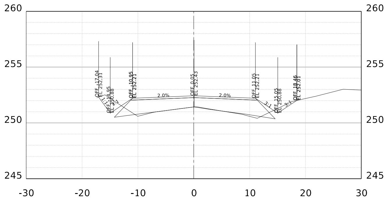
STA. 76+00.00 R1
