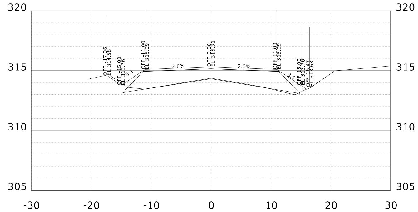
STA. 4+00.00 R1
