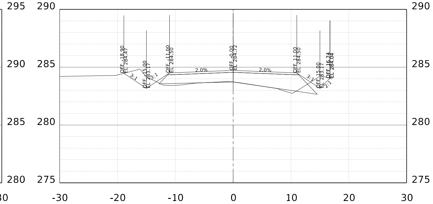
STA. 115+00.00 R1
