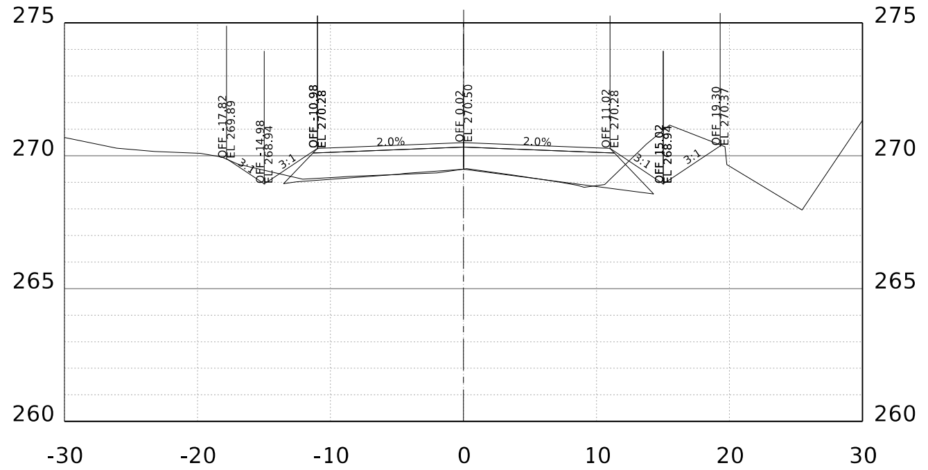
STA. 147+00.00 R1
