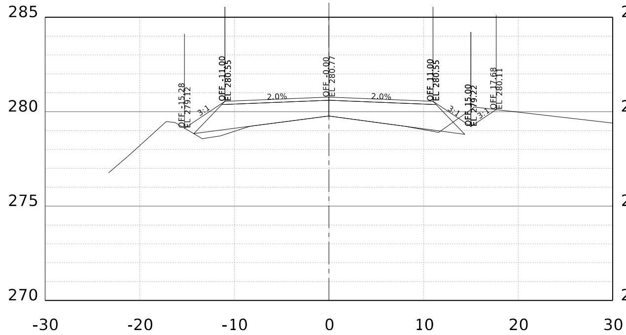
STA. 133+00.00 R1
