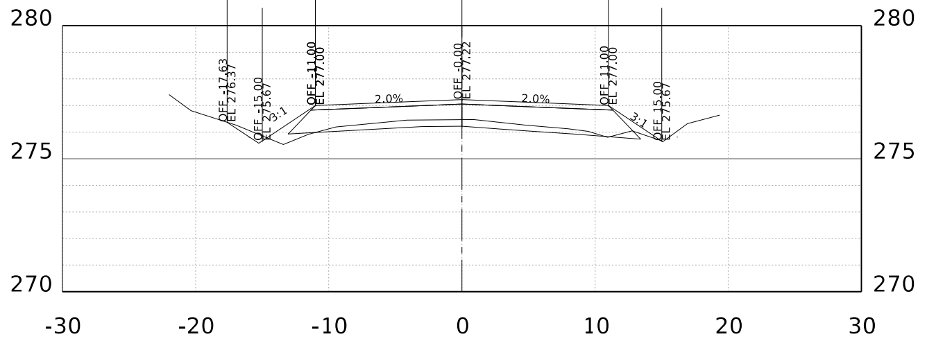
STA. 48+00.00 R1
