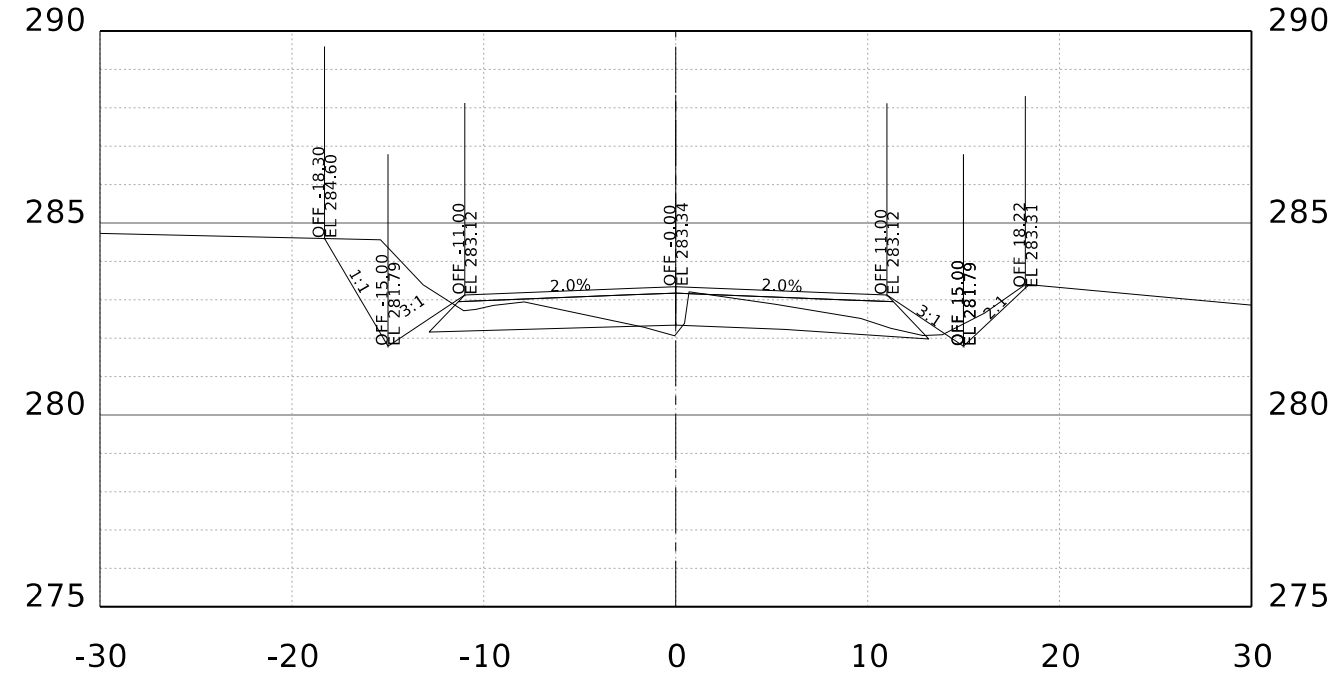
STA. 103+00.00 R1
