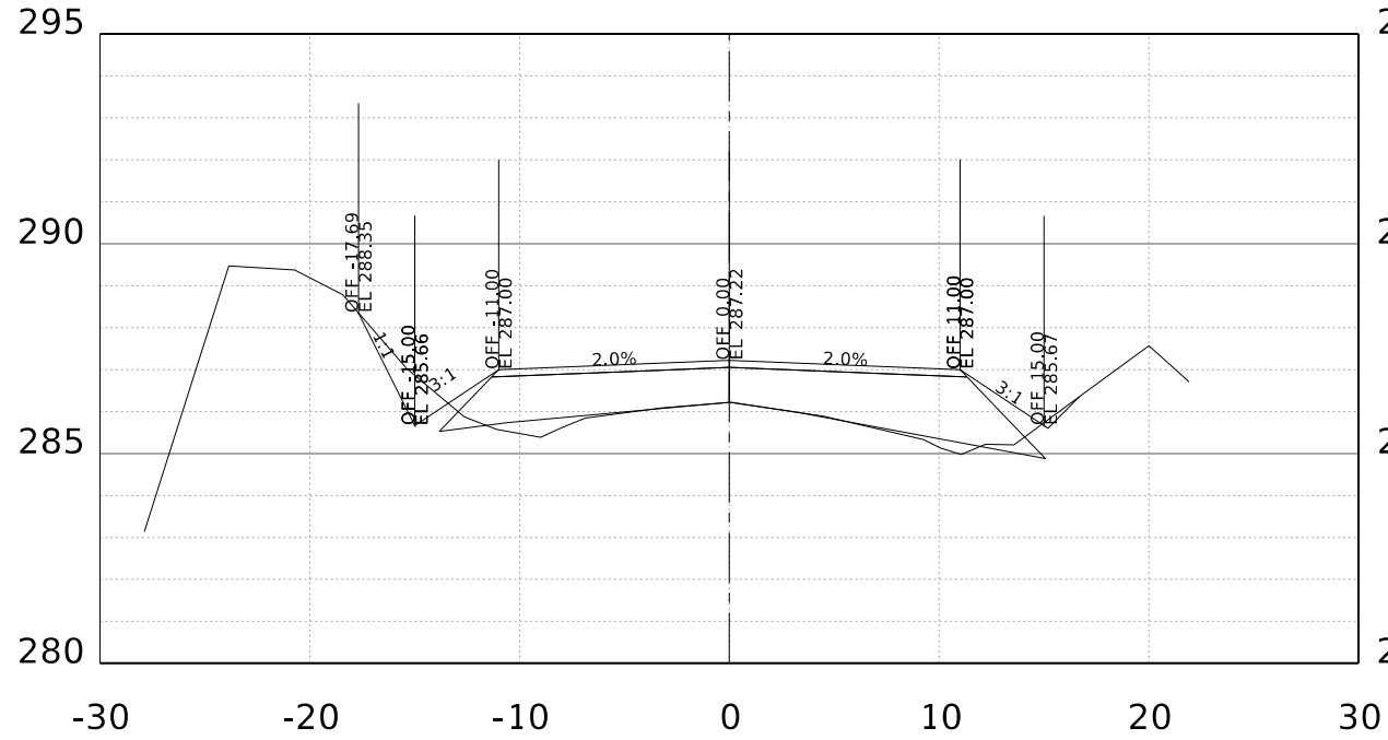
STA. 39+00.00 R1
