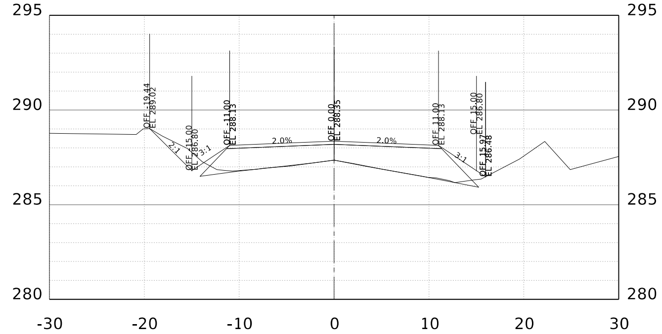
STA. 26+00.00 R1
