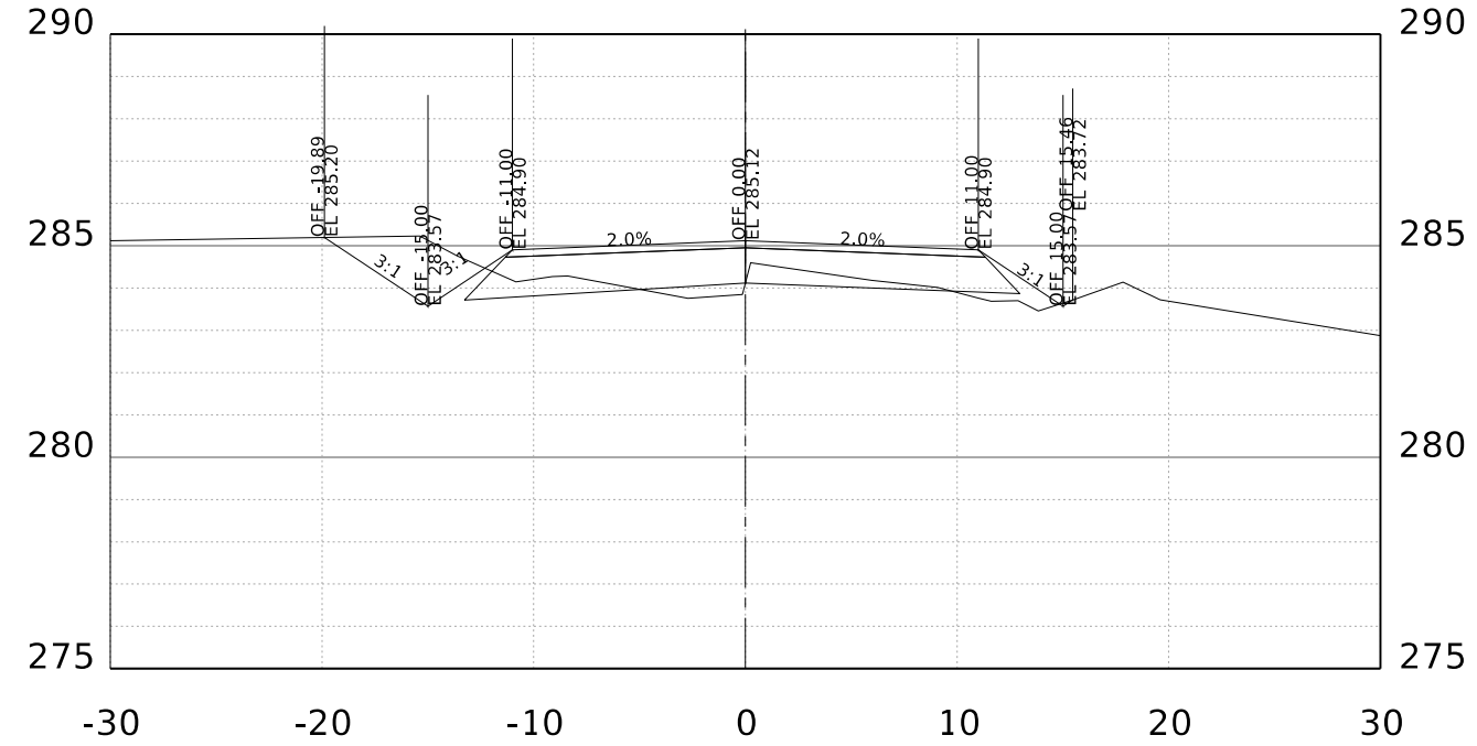
STA. 105+00.00 R1
