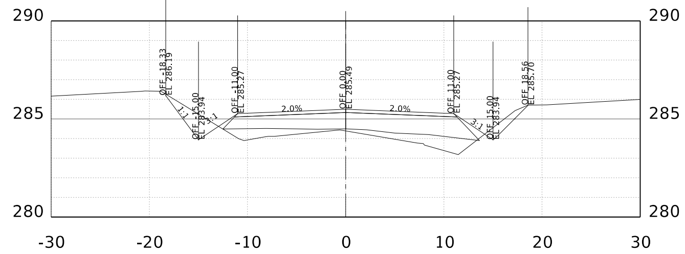
STA. 17+00.00 R1
