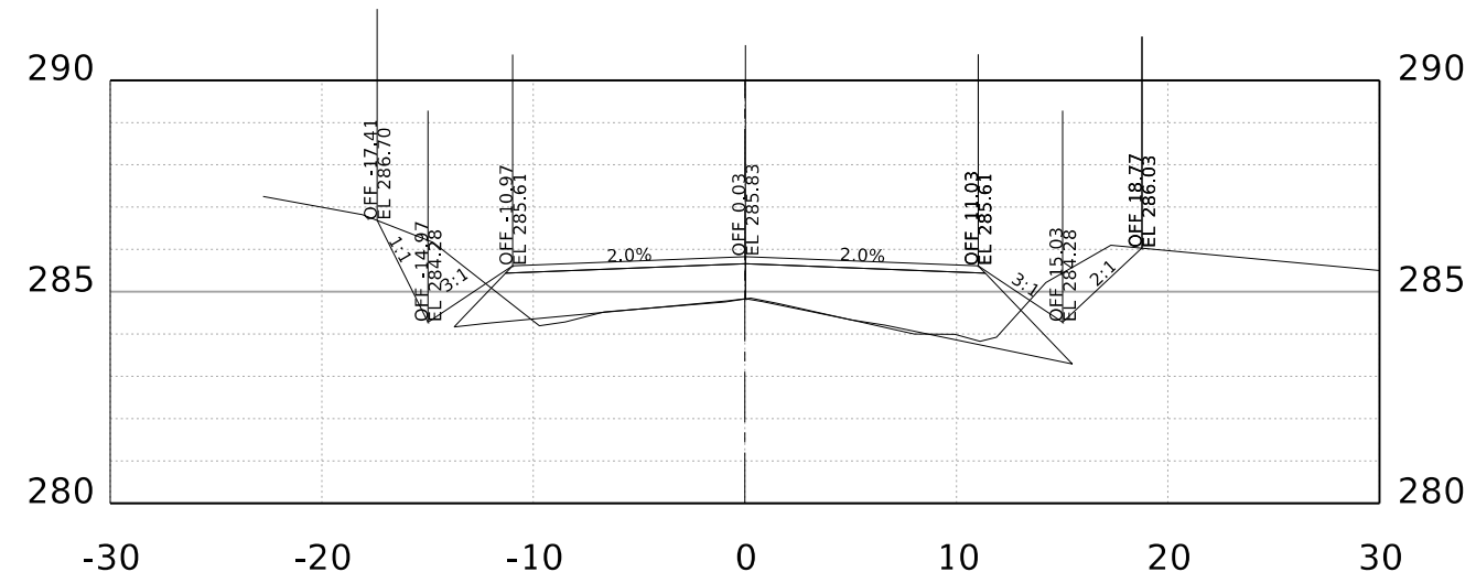
STA. 24+00.00 R1
