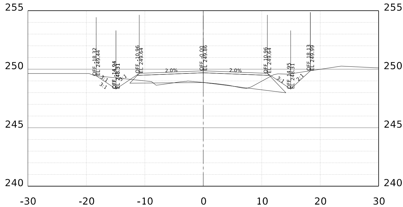
STA. 73+00.00 R1
