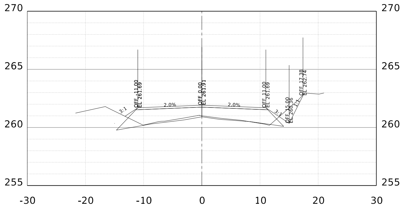
STA. 82+00.00 R1
