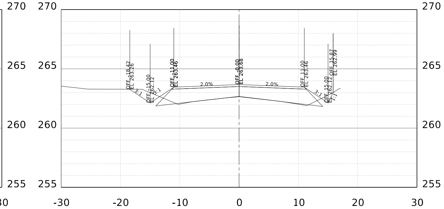
STA. 84+00.00 R1
