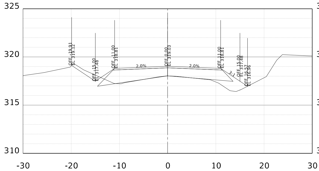
STA. 2+00.00 R1
