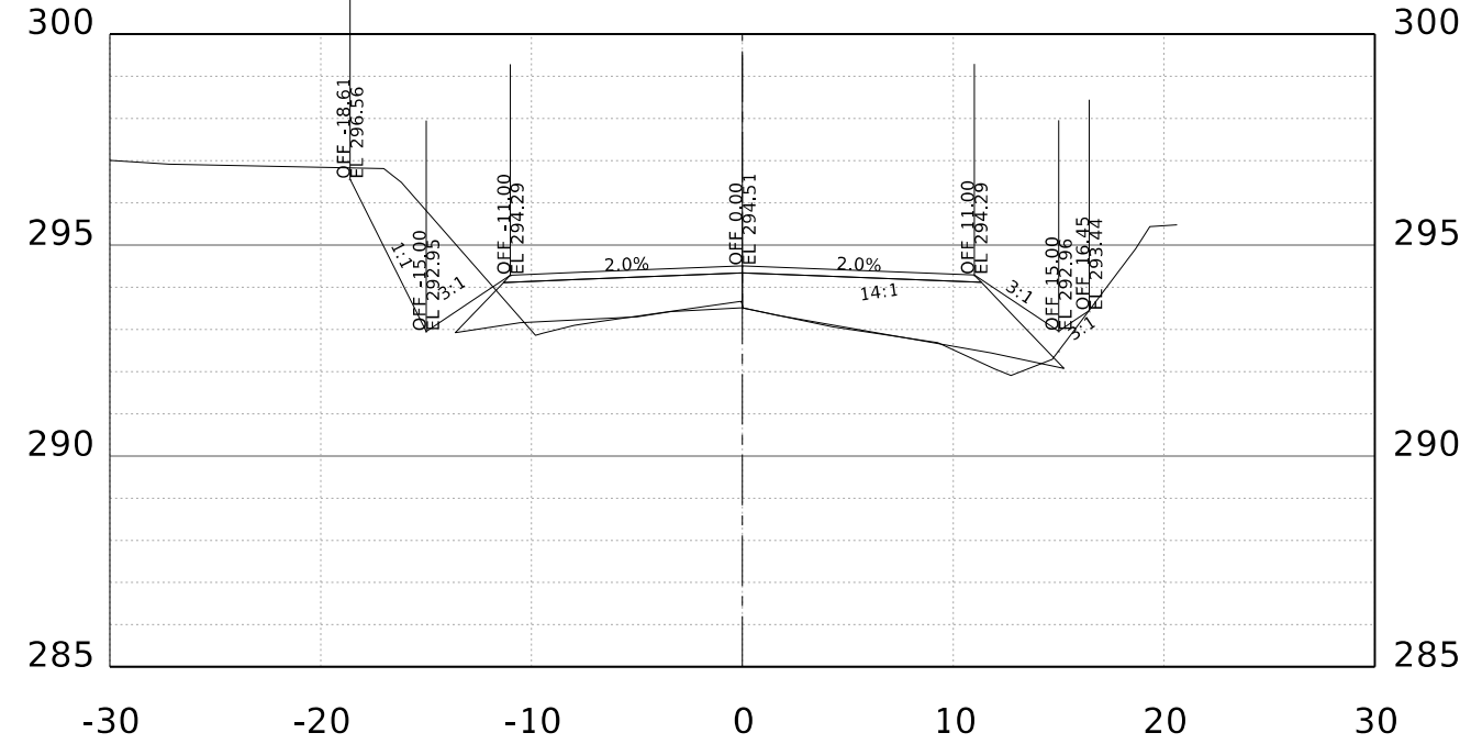
STA. 14+00.00 R1
