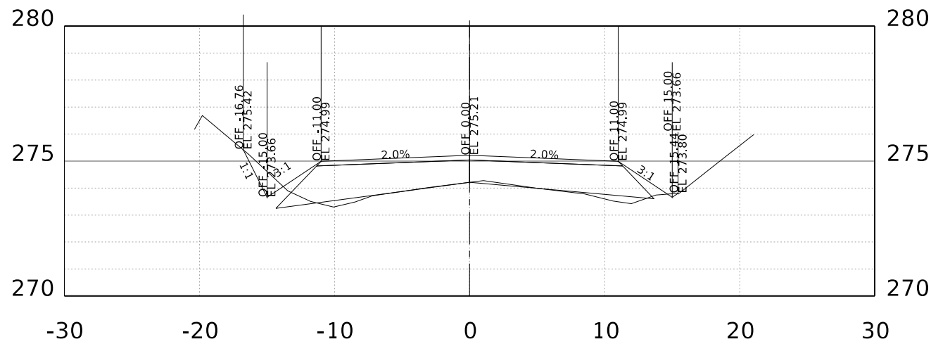
STA. 50+00.00 R1
