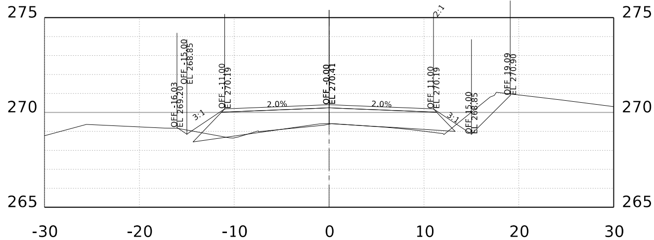
STA. 91+00.00 R1
