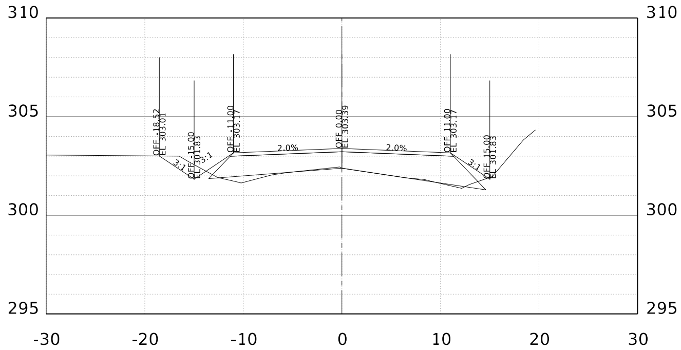
STA. 10+00.00 R1
