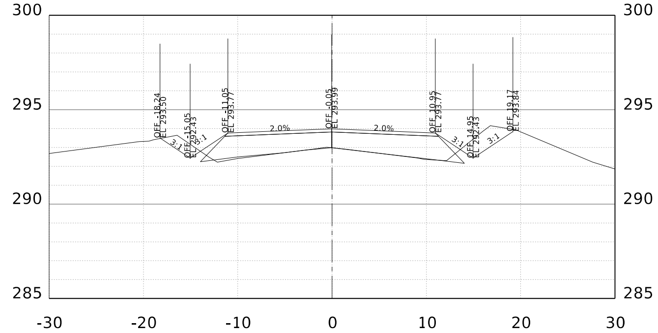
STA. 111+00.00 R1
