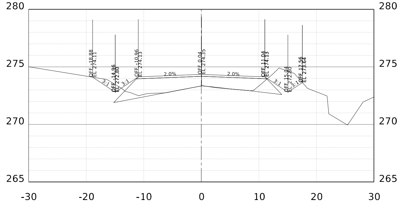
STA. 148+00.00 R1
