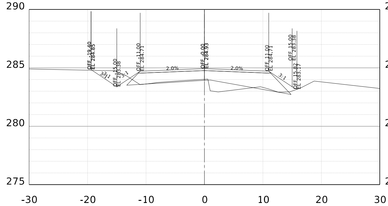
STA. 104+00.00 R1
