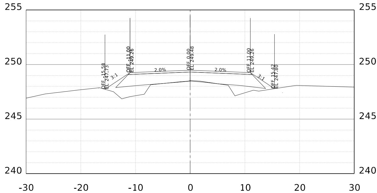
STA. 71+00.00 R1
