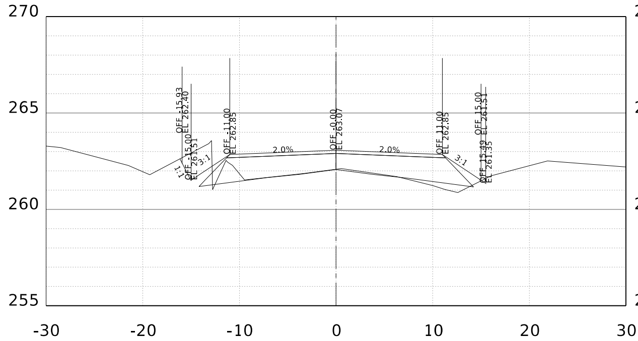
STA. 59+00.00 R1
