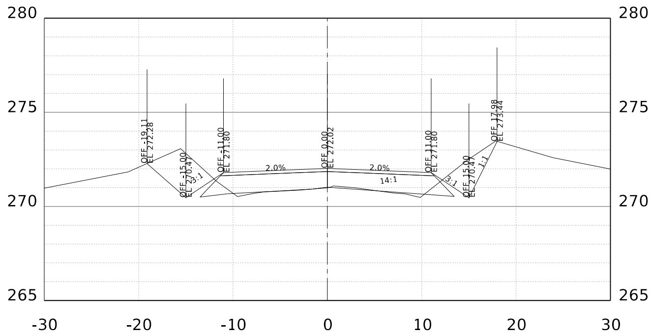
STA. 94+00.00 R1
