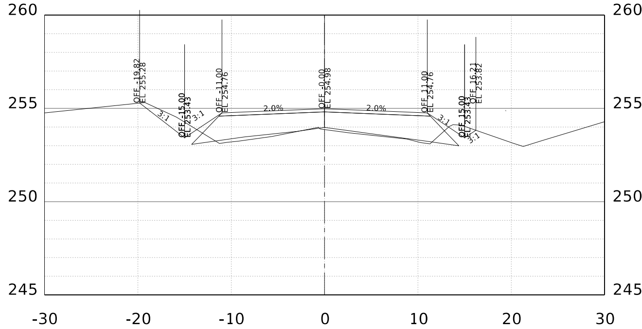
STA. 63+00.00 R1
