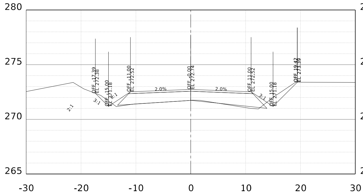
STA. 95+00.00 R1
