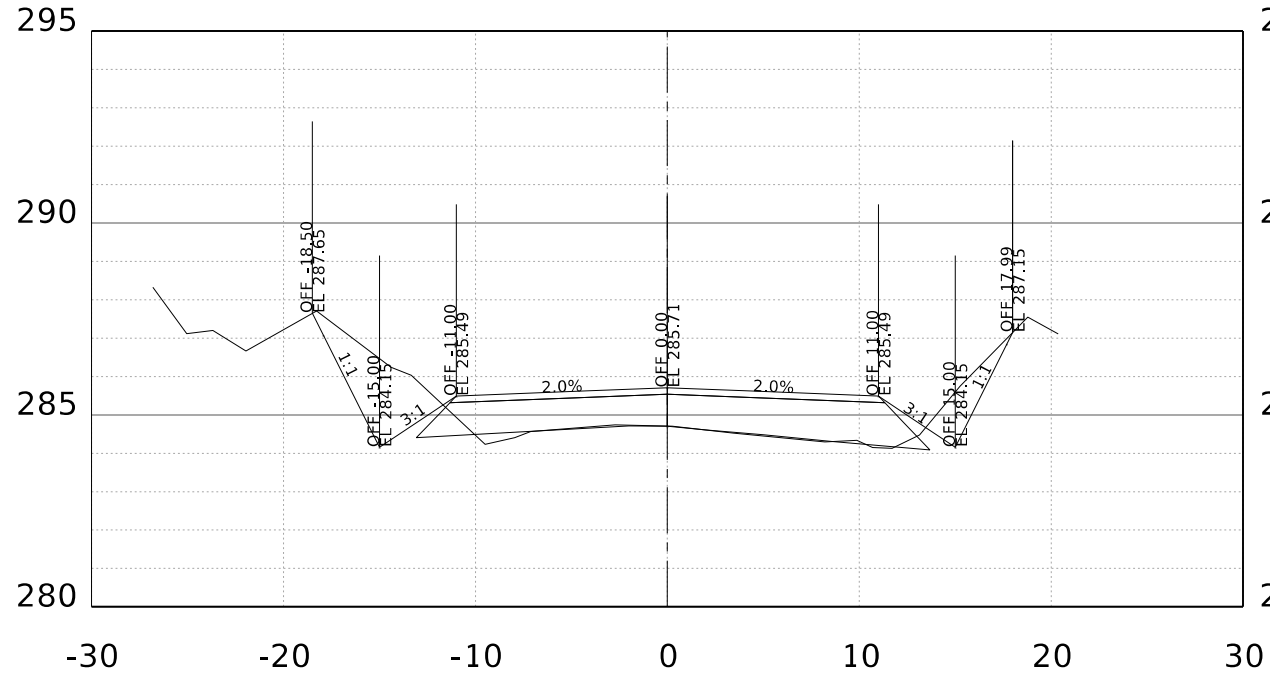
STA. 33+00.00 R1
