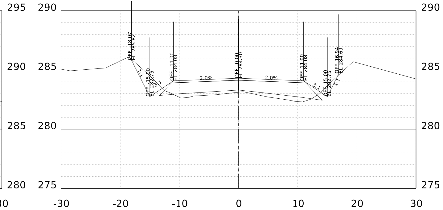
STA. 28+00.00 R1
