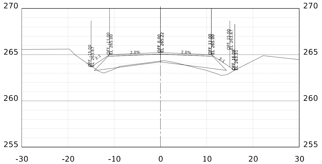
STA. 58+00.00 R1
