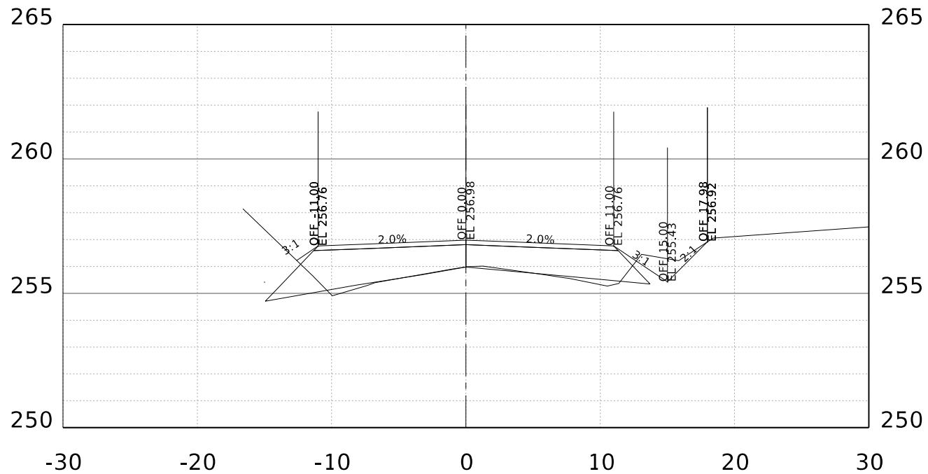
STA. 79+00.00 R1
