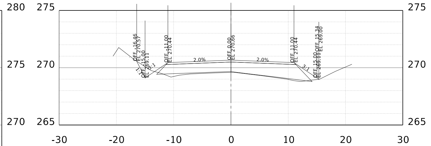
STA. 53+00.00 R1
