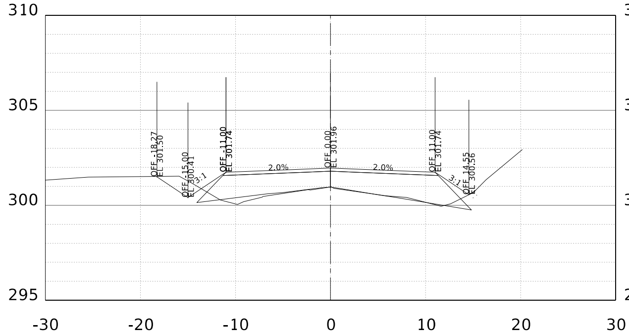
STA. 11+00.00 R1
