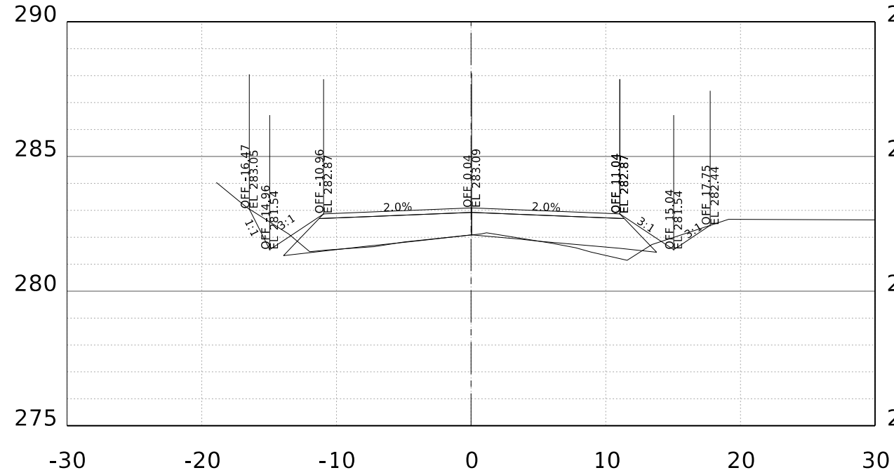
STA. 22+00.00 R1
