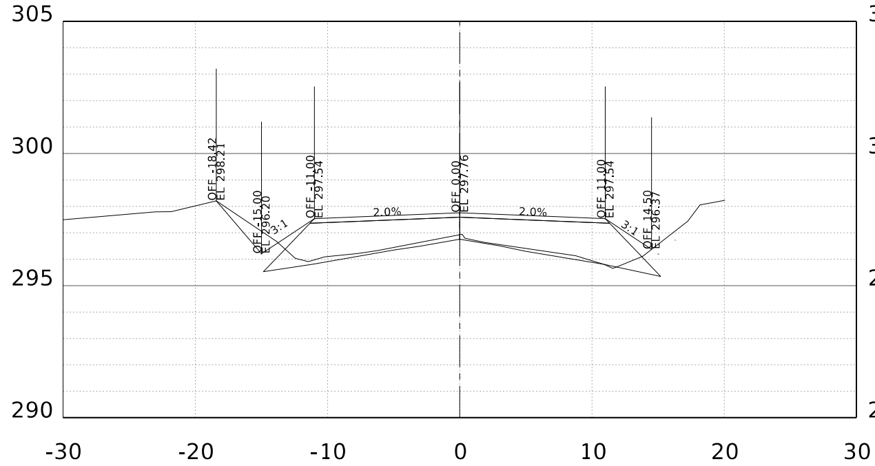
STA. 13+00.00 R1
