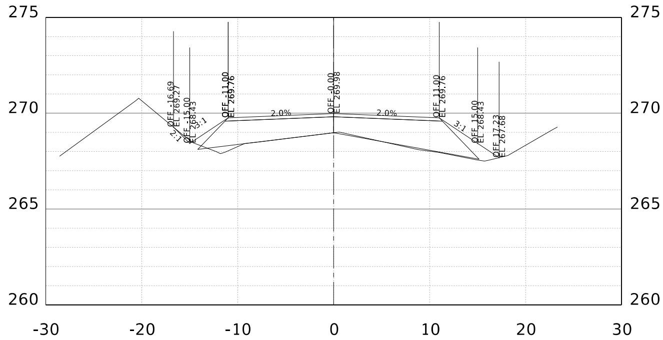
STA. 55+00.00 R1
