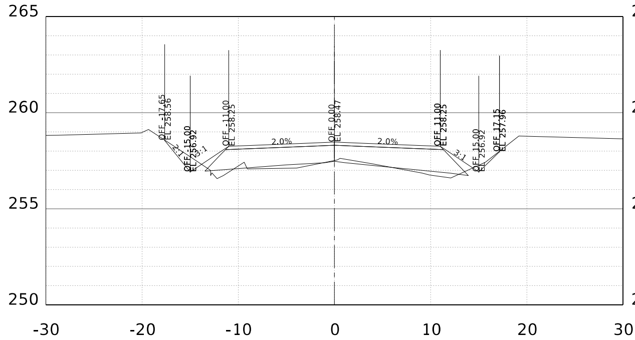
STA. 61+00.00 R1
