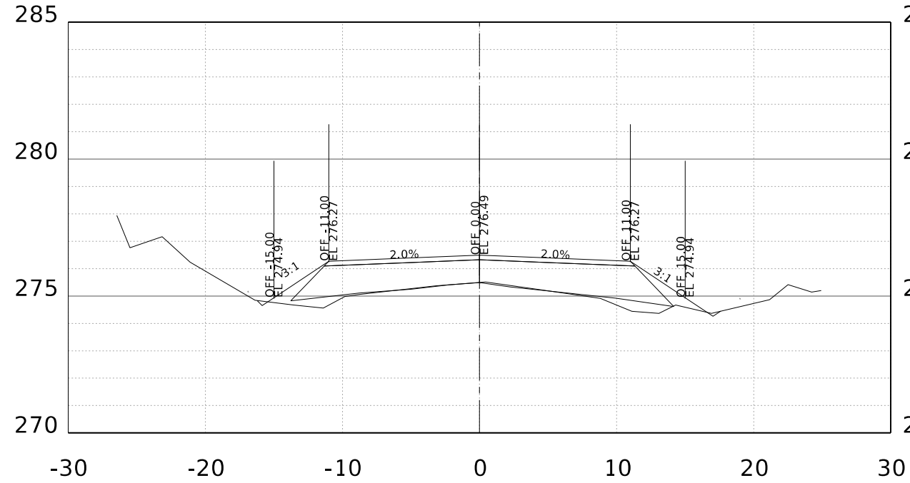
STA. 43+00.00 R1
