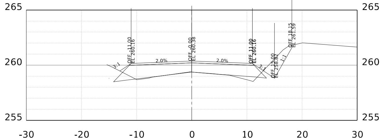
STA. 81+00.00 R1
