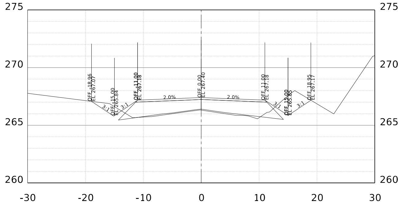
STA. 146+00.00 R1
