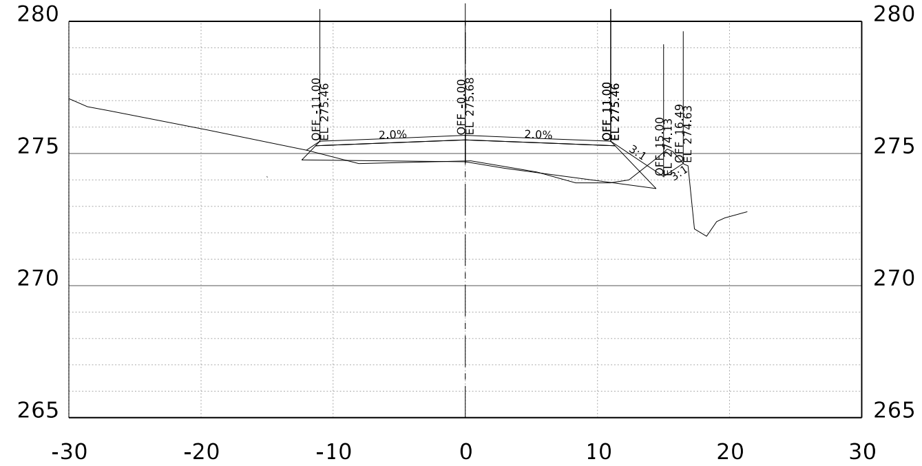
STA. 149+00.00 R1
