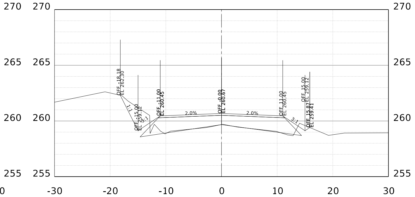
STA. 60+00.00 R1
