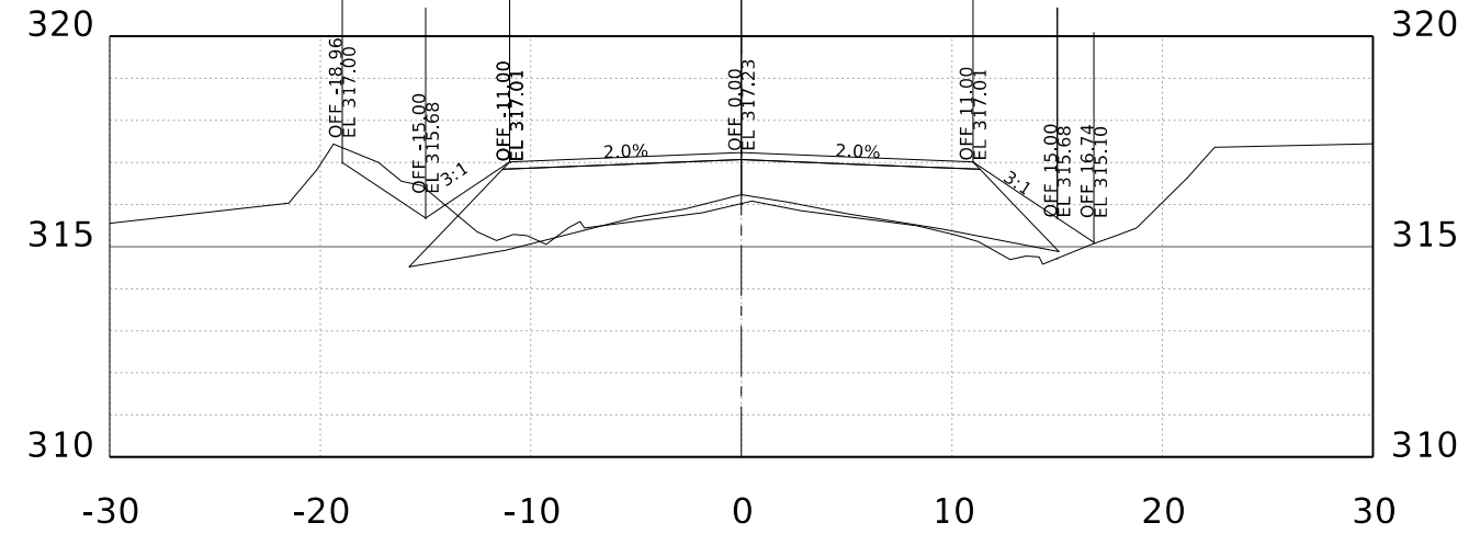
STA. 3+00.00 R1
