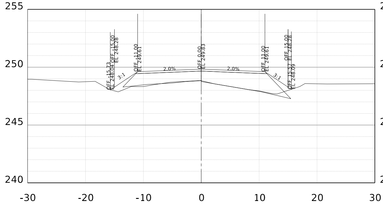
STA. 69+00.00 R1
