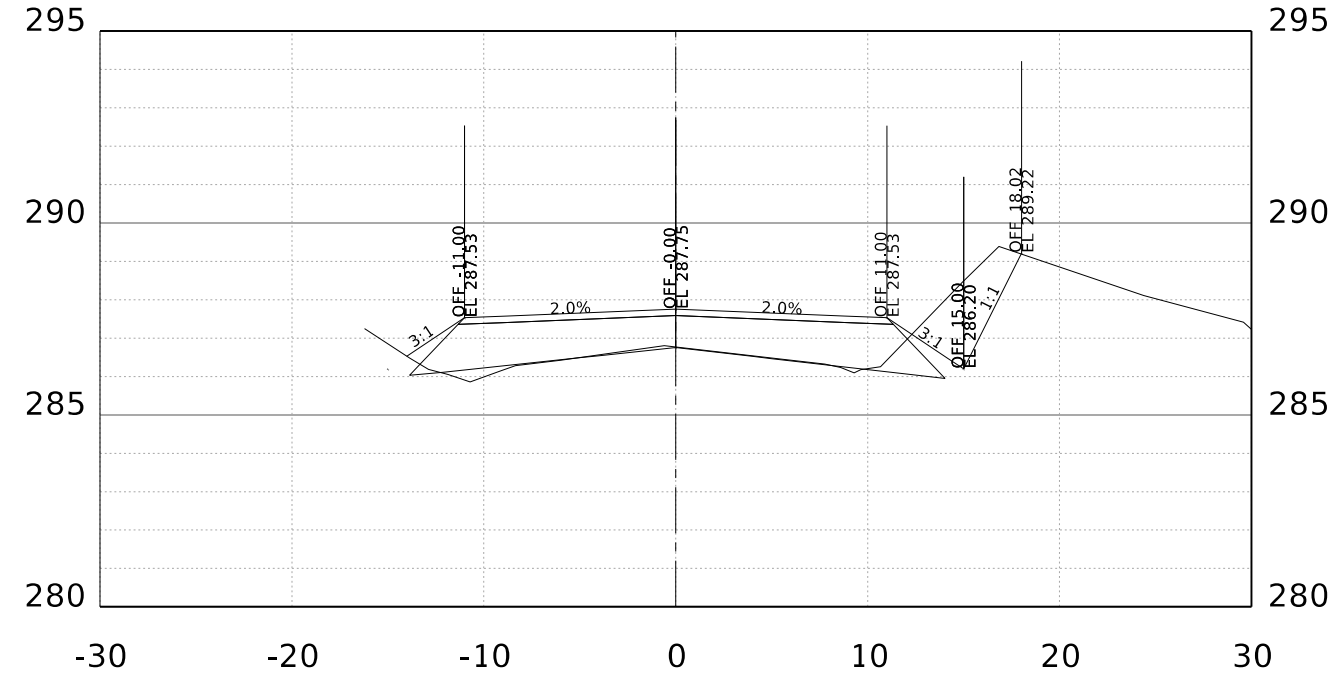
STA. 129+00.00 R1
