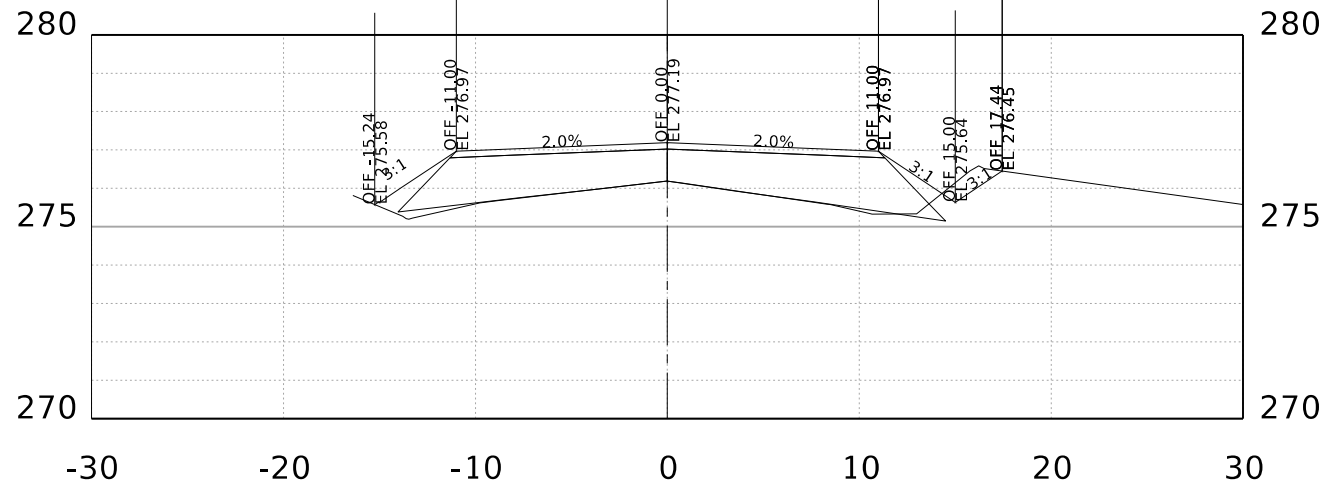
STA. 136+00.00 R1
