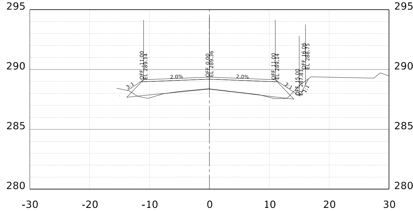
STA. 128+00.00 R1
