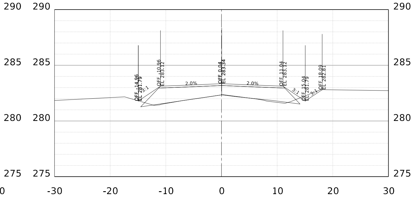
STA. 19+00.00 R1
