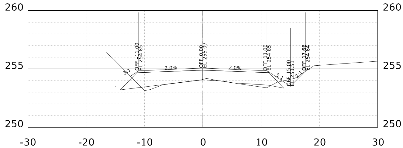
STA. 78+00.00 R1
