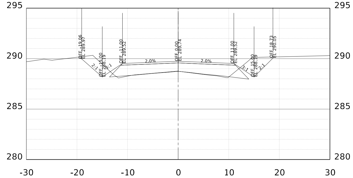
STA. 108+00.00 R1
