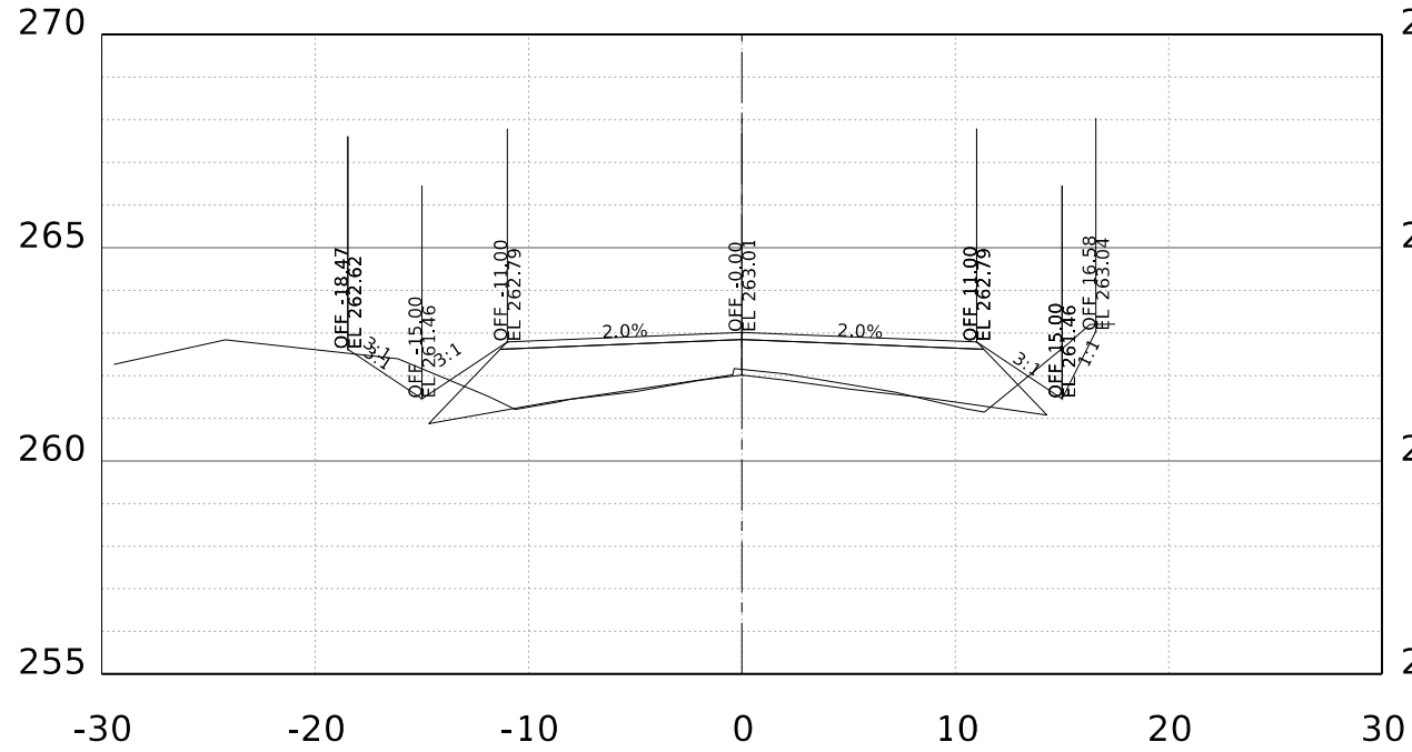
STA. 83+00.00 R1
