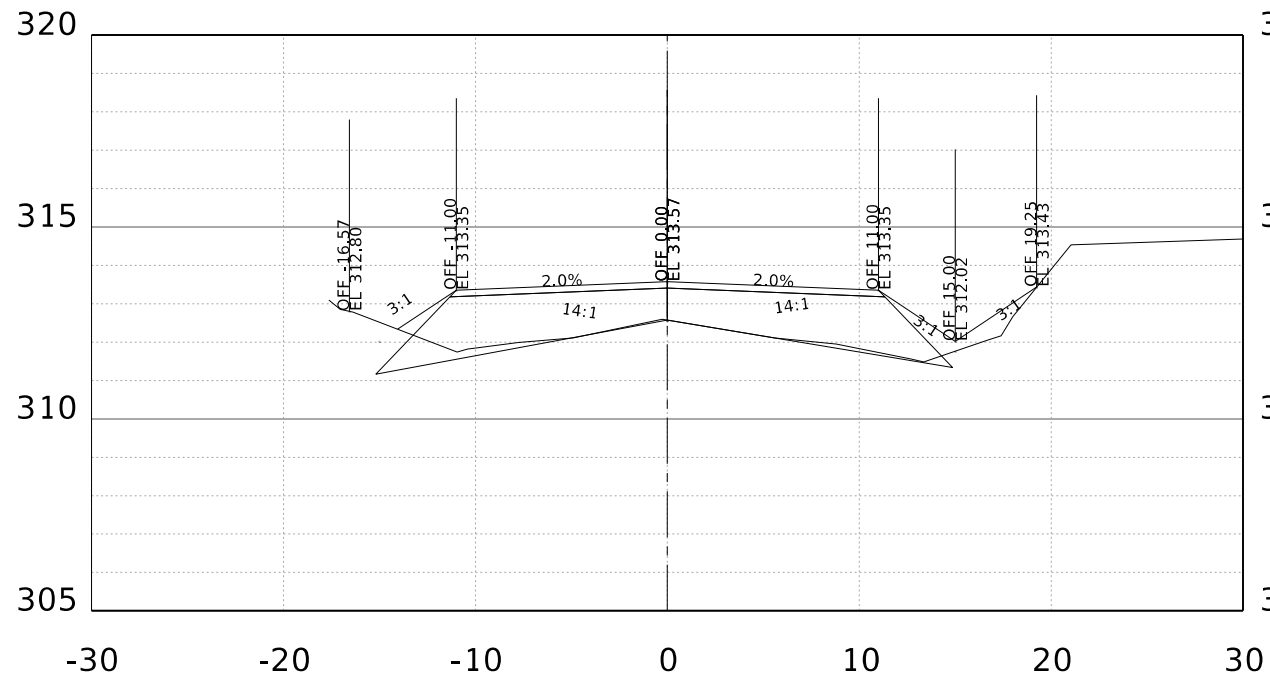
STA. 5+00.00 R1
