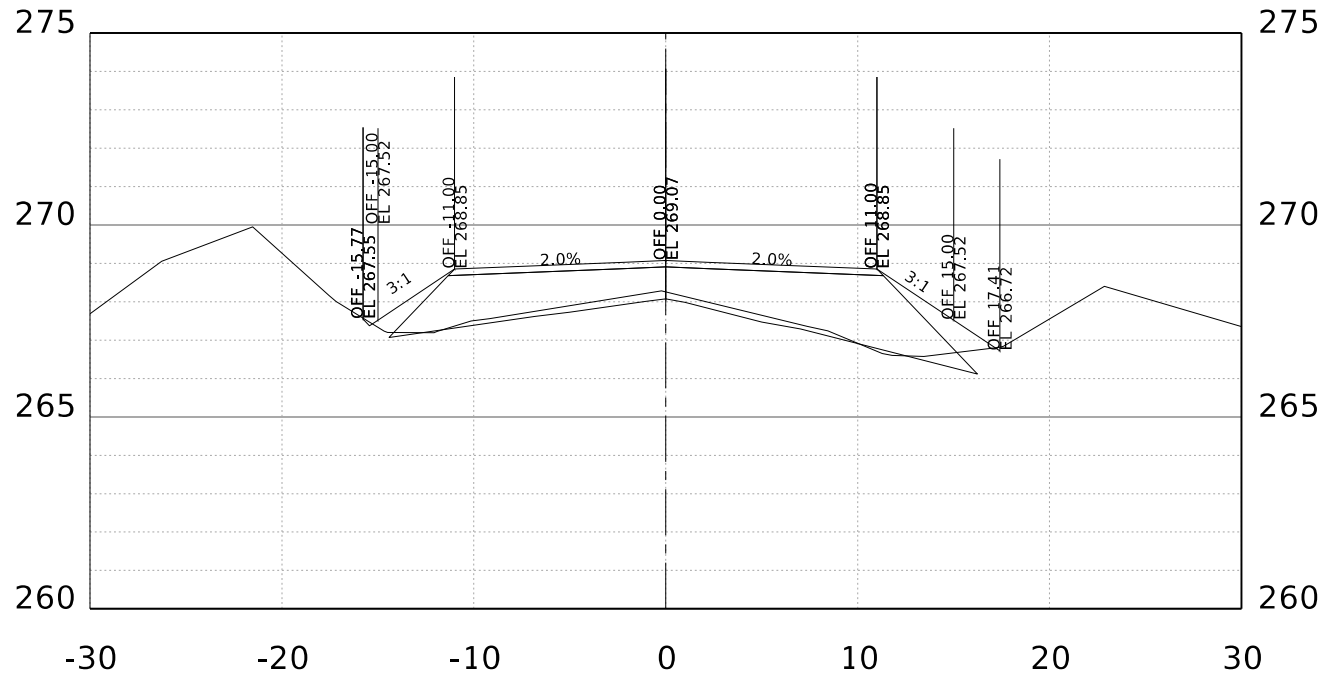
STA. 56+00.00 R1
