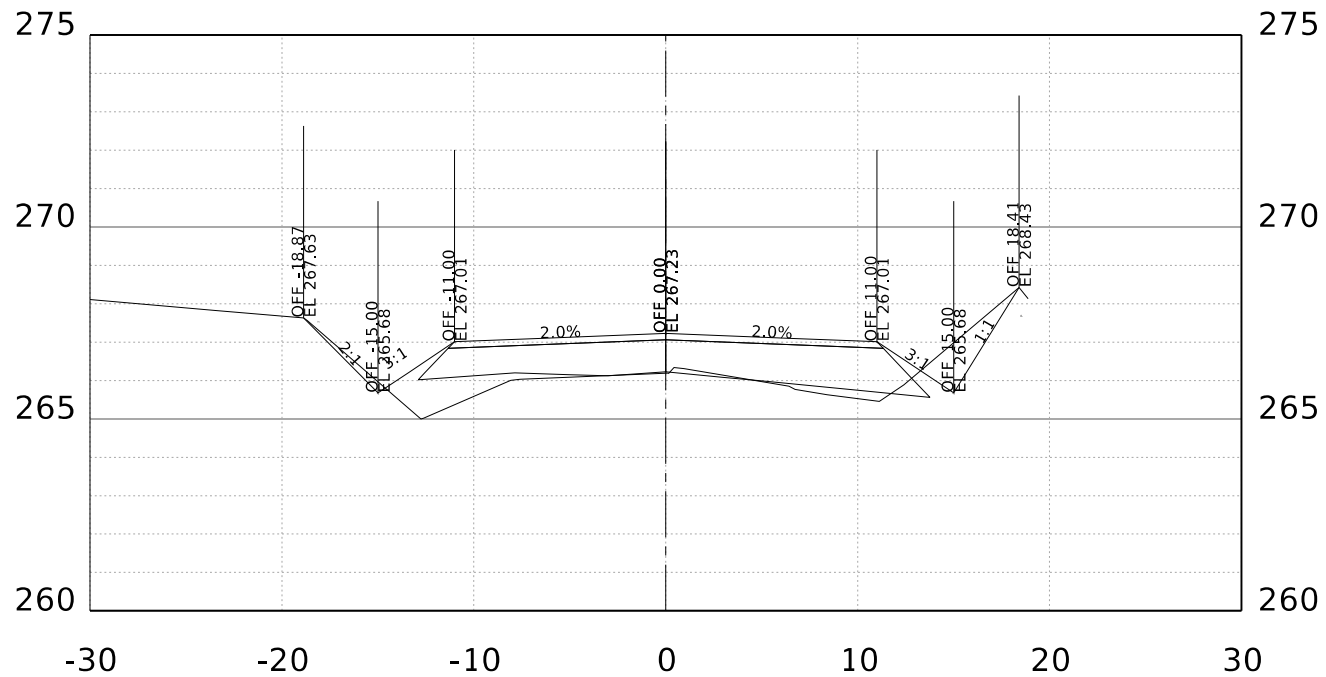
STA. 87+00.00 R1
