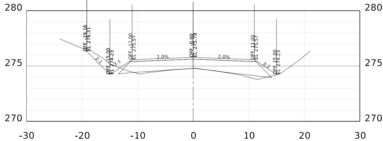
STA. 46+00.00 R1
