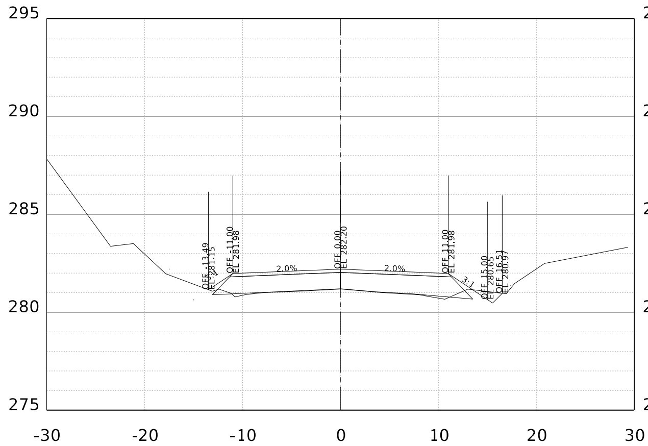
STA. 31+00.00 R1
