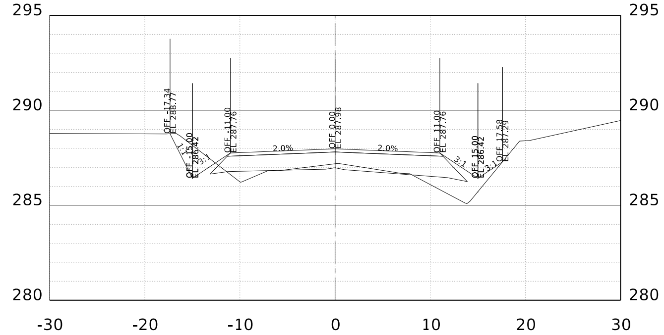
STA. 16+00.00 R1
