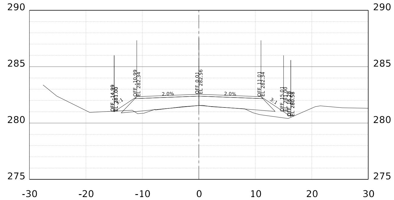
STA. 21+00.00 R1
