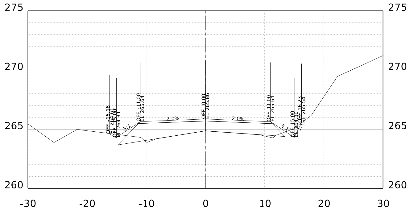
STA. 143+00.00 R1
