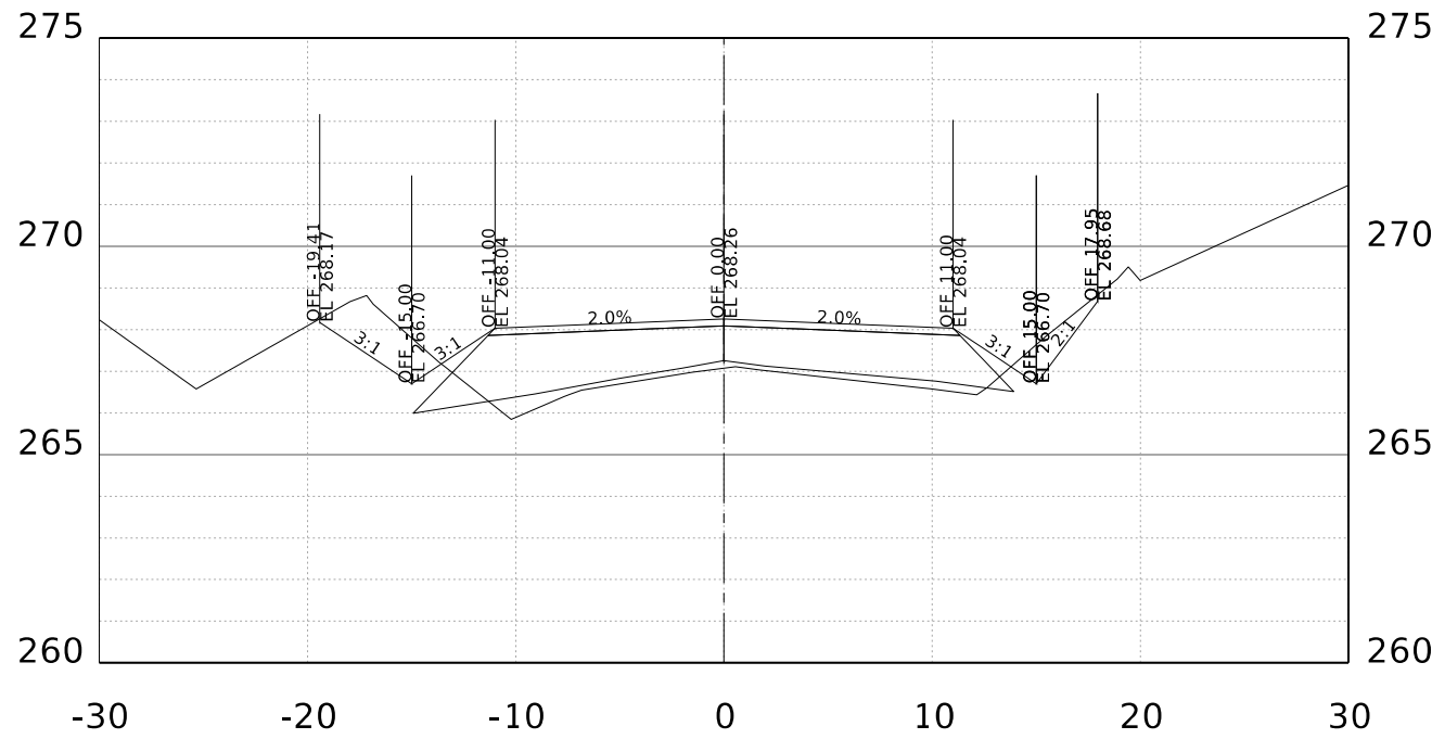
STA. 142+00.00 R1
