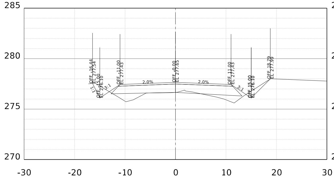
STA. 100+00.00 R1
