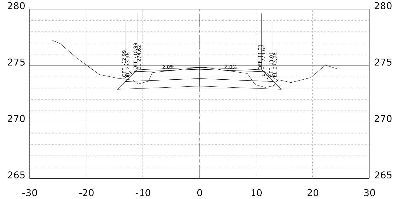
STA. 44+00.00 R1
