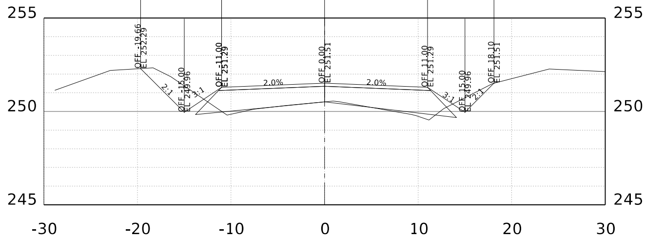
STA. 75+00.00 R1
