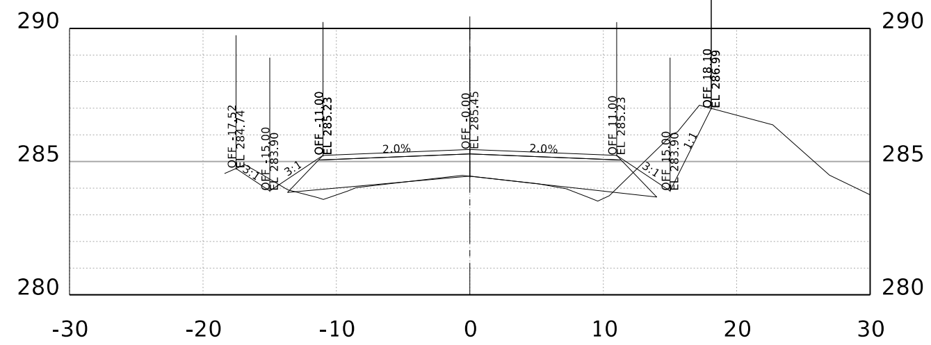
STA. 130+00.00 R1
