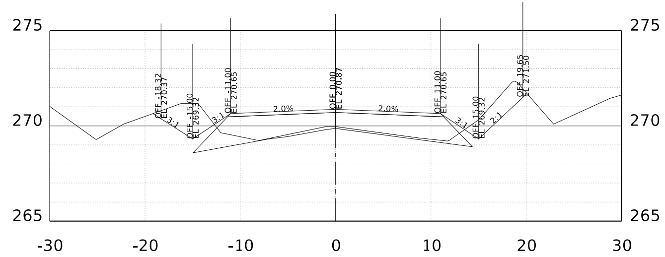
STA. 141+00.00 R1
