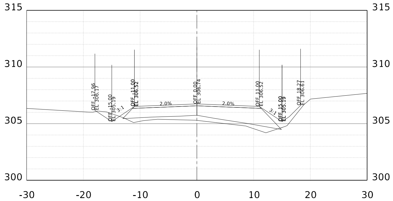
STA. 8+00.00 R1
