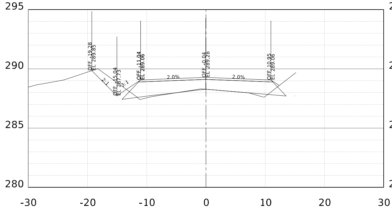
STA. 114+00.00 R1
