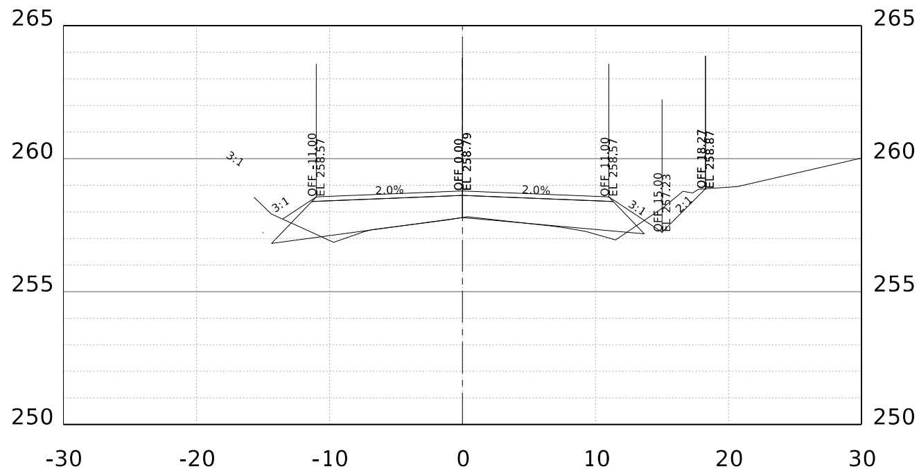
STA. 80+00.00 R1
