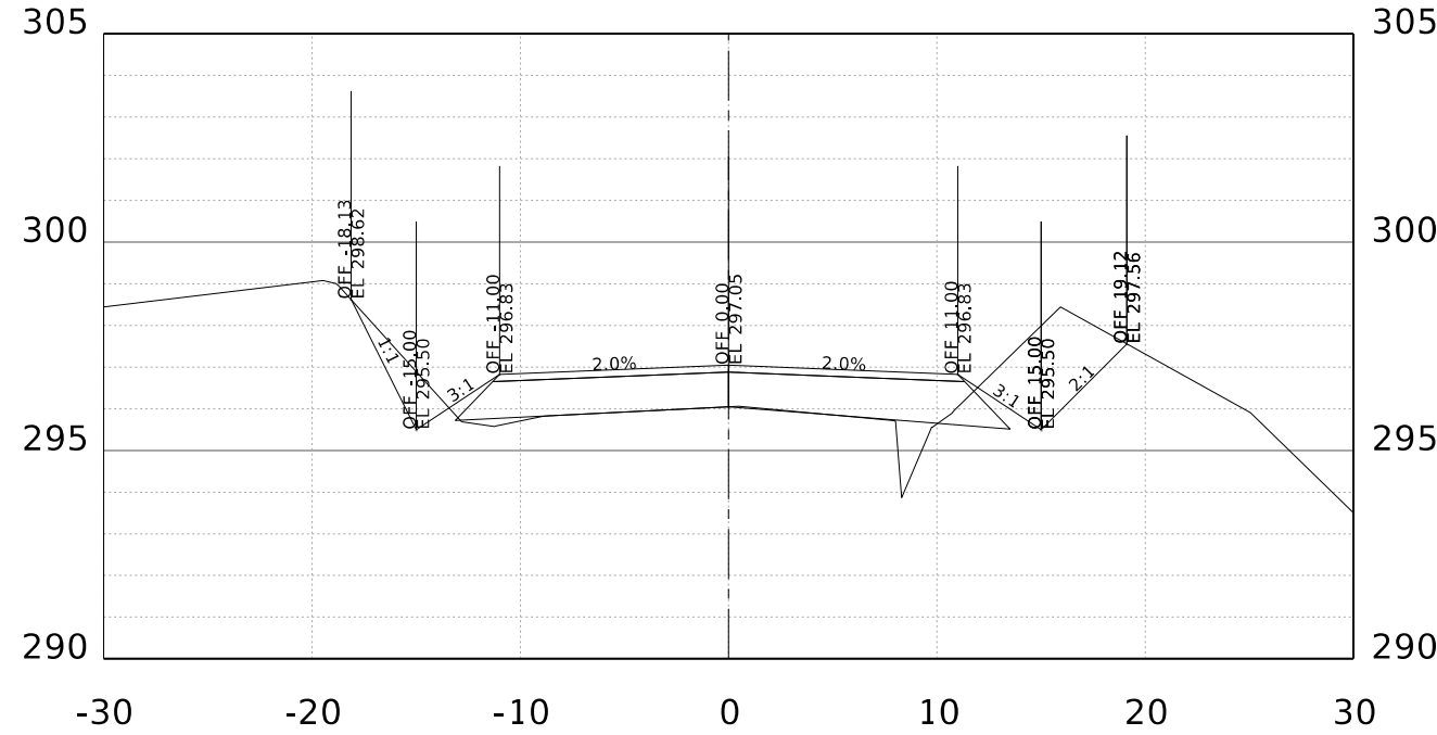
STA. 125+00.00 R1
