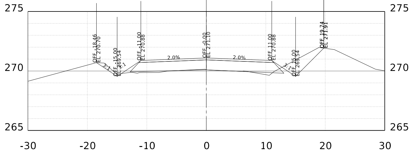
STA. 90+00.00 R1
