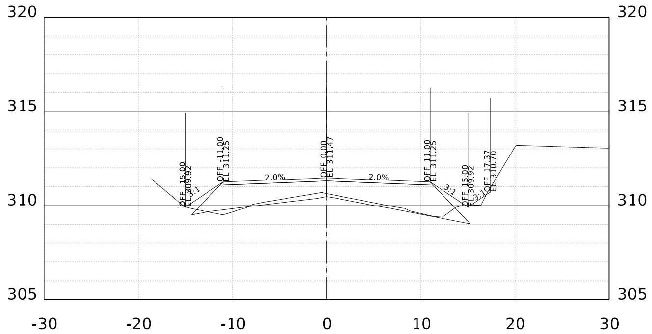
STA. 6+00.00 R1
