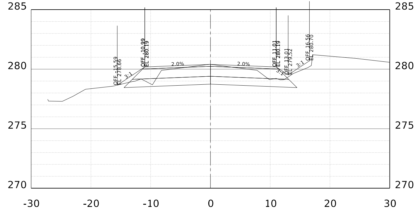
STA. 132+00.00 R1
