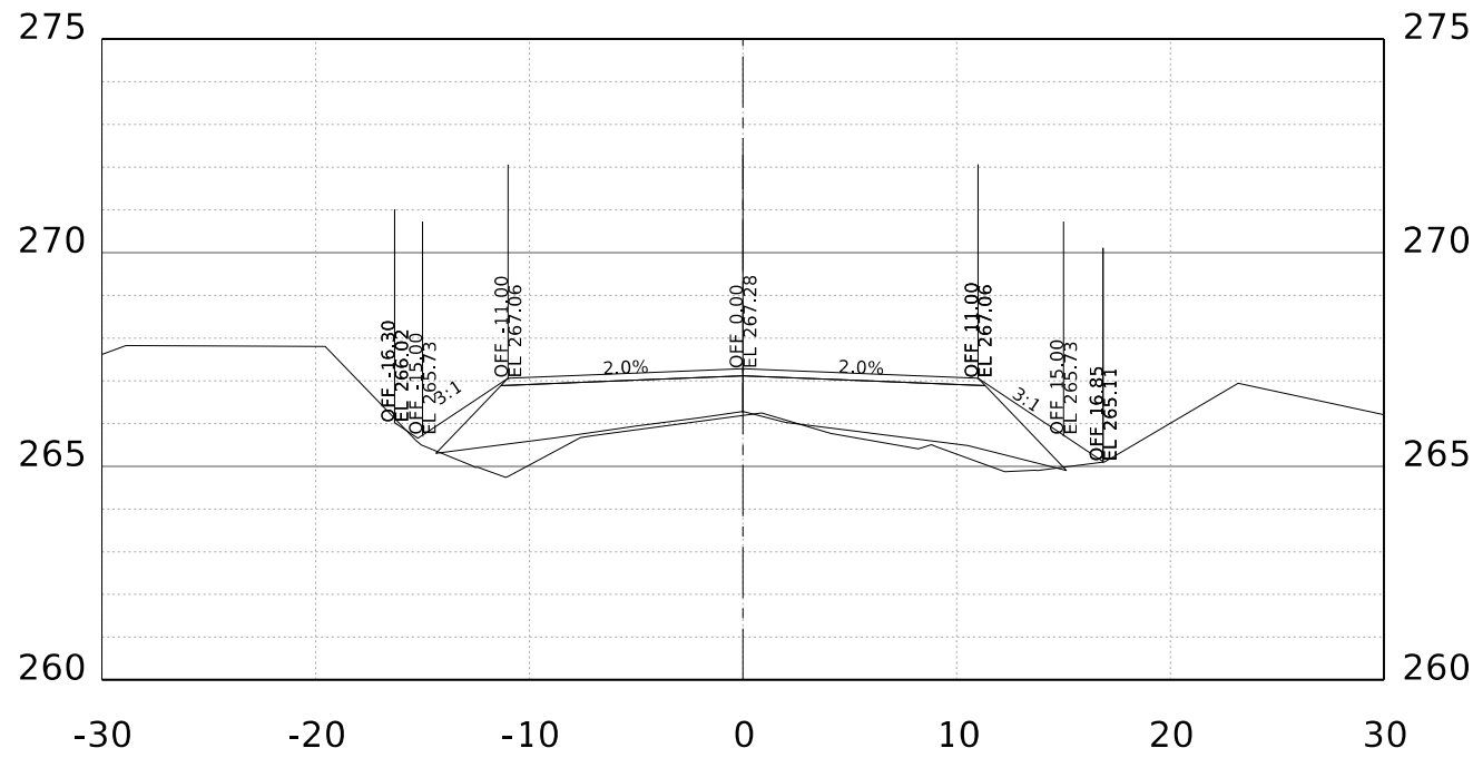
STA. 57+00.00 R1
