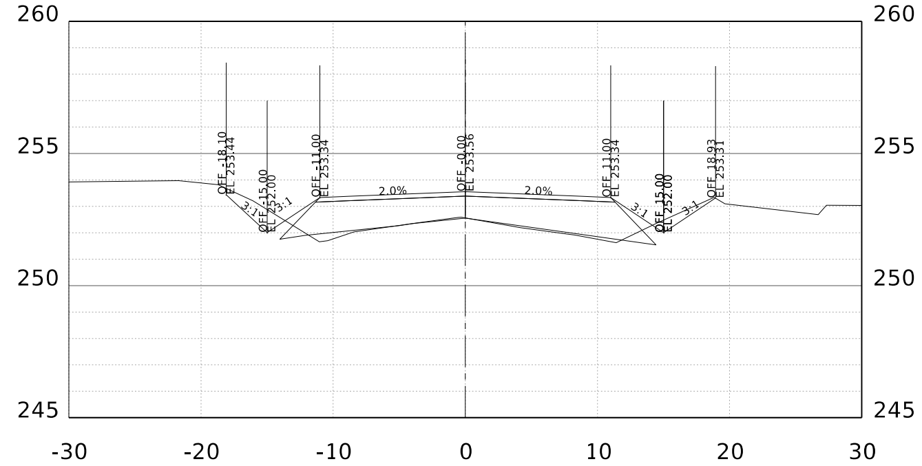
STA. 64+00.00 R1
