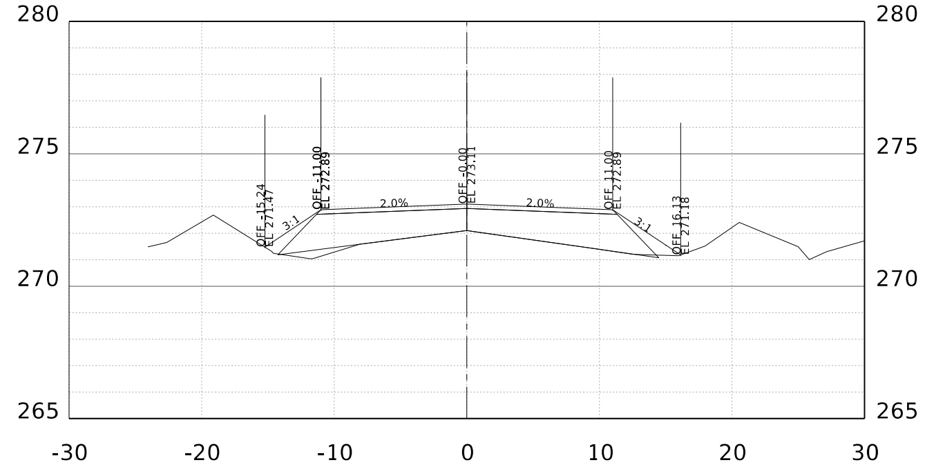
STA. 140+00.00 R1
