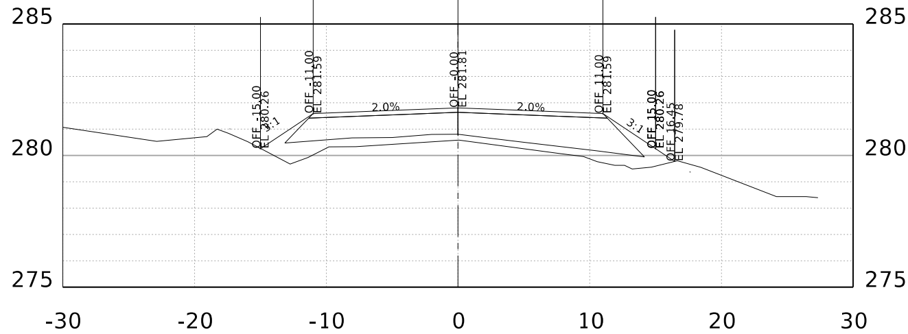
STA. 117+00.00 R1
