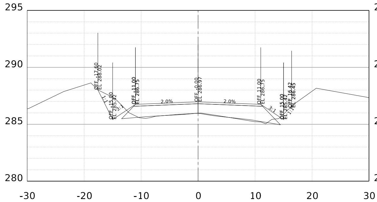
STA. 27+00.00 R1
