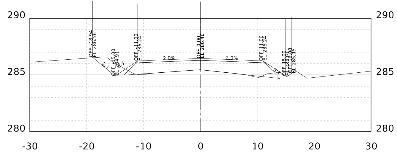
STA. 106+00.00 R1
