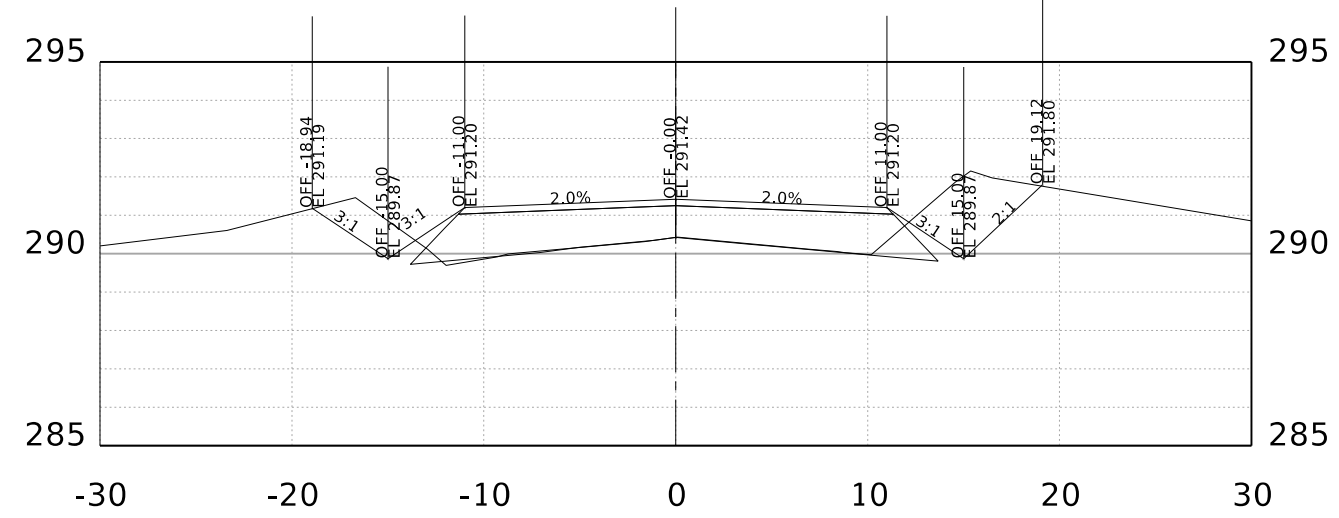
STA. 109+00.00 R1
