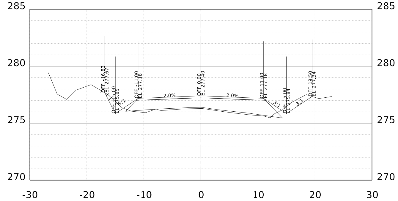
STA. 42+00.00 R1
