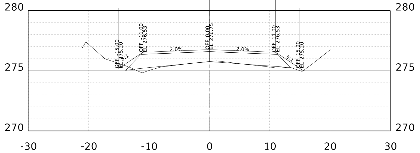
STA. 49+00.00 R1
