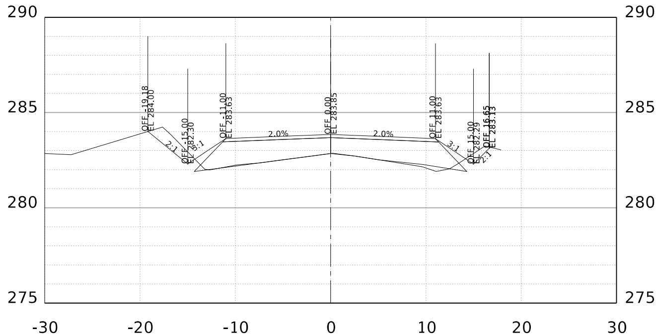
STA. 119+00.00 R1
