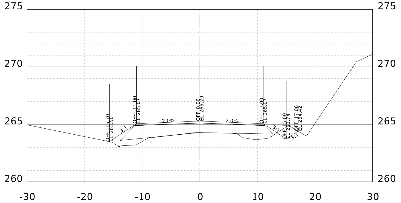
STA. 145+00.00 R1
