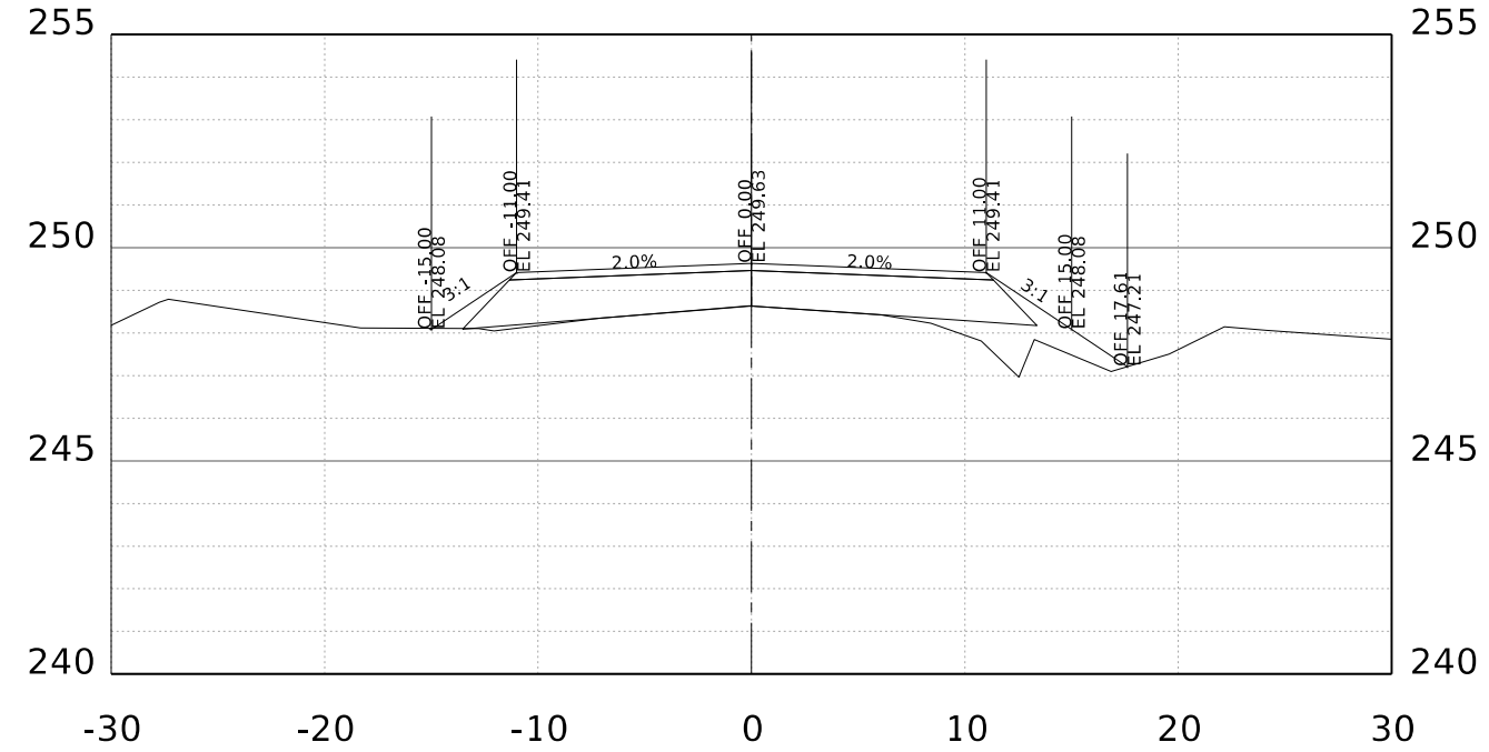
STA. 70+00.00 R1
