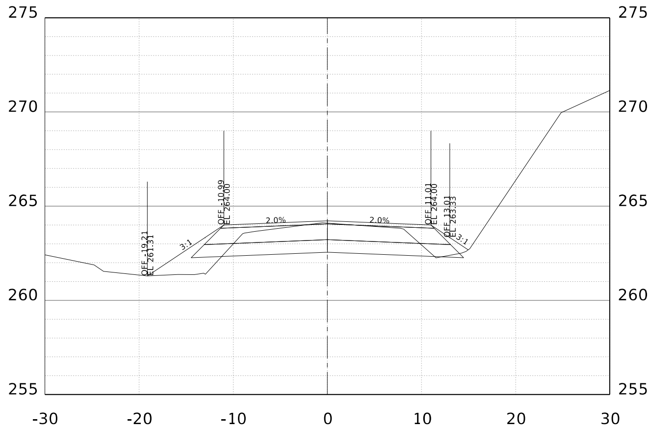
STA. 144+00.00 R1
