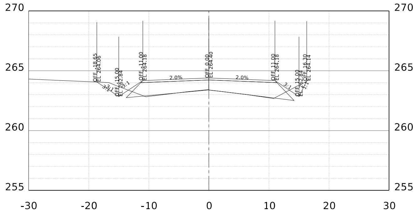
STA. 85+00.00 R1
