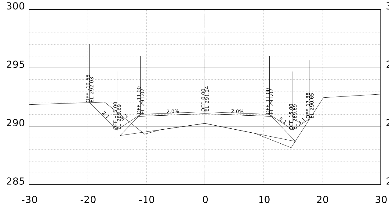
STA. 15+00.00 R1
