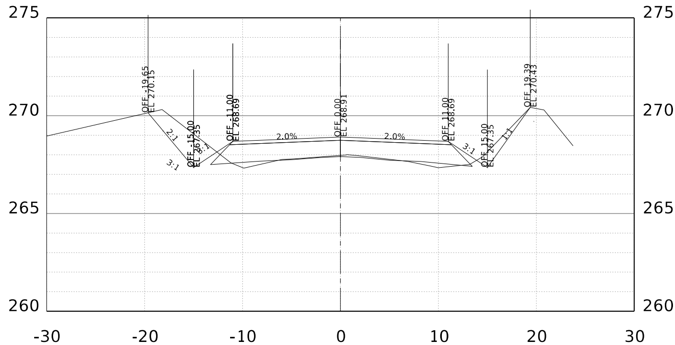
STA. 88+00.00 R1
