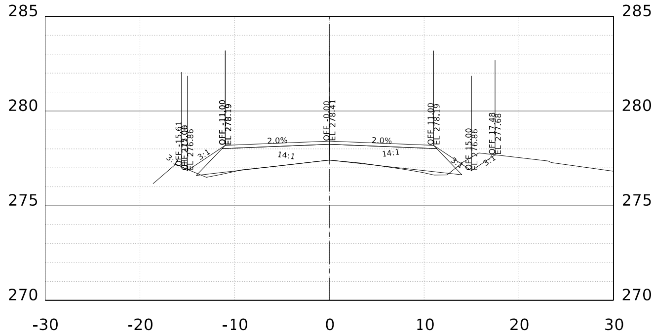
STA. 135+00.00 R1
