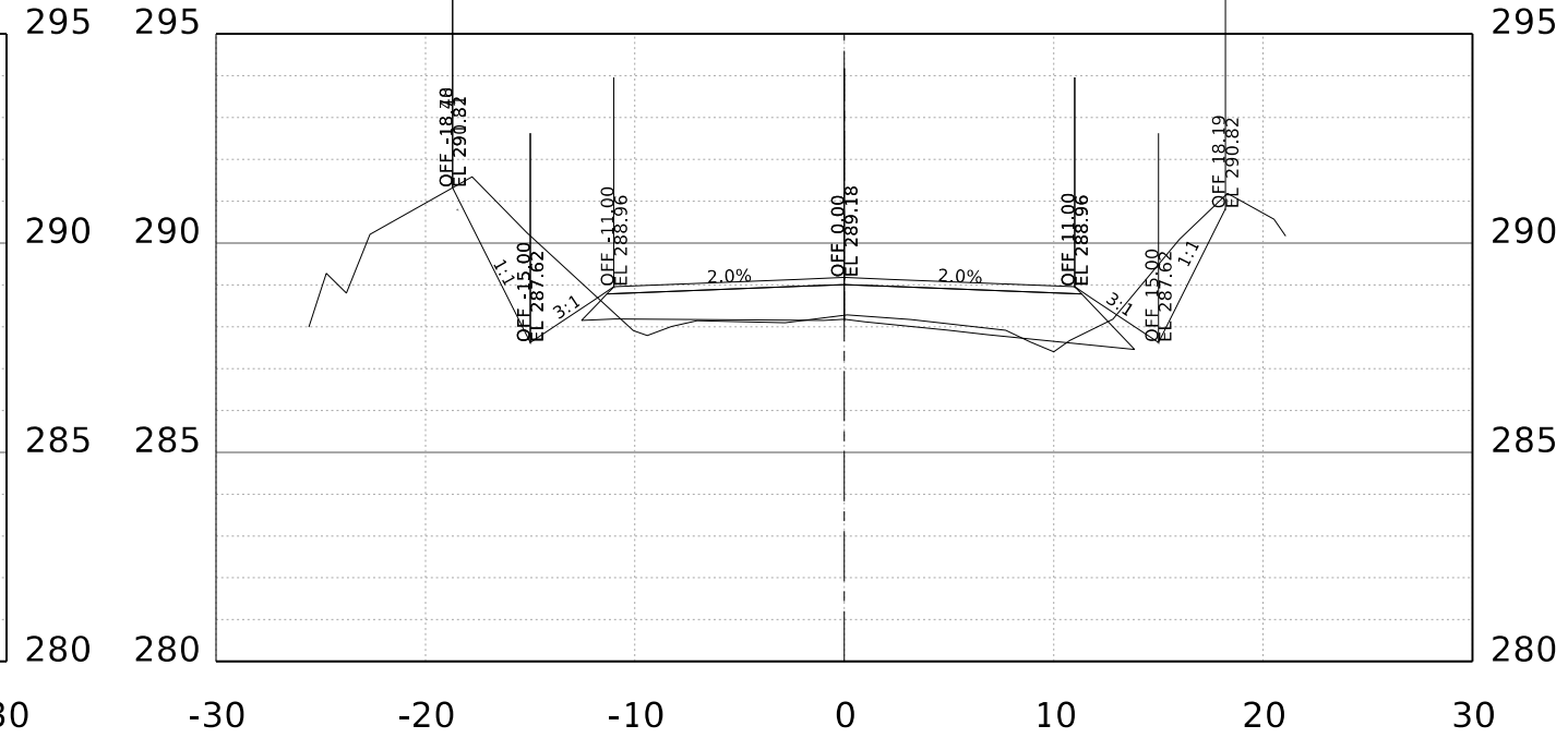
STA. 34+00.00 R1
