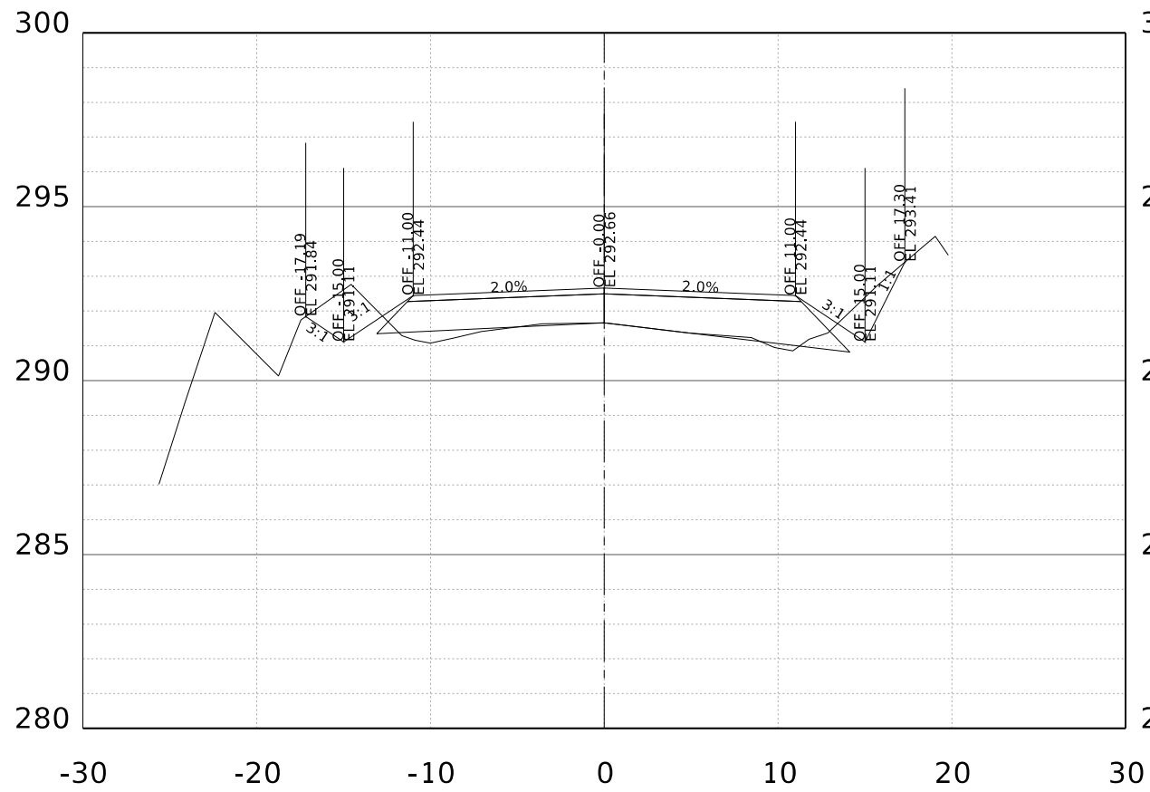
STA. 35+00.00 R1
