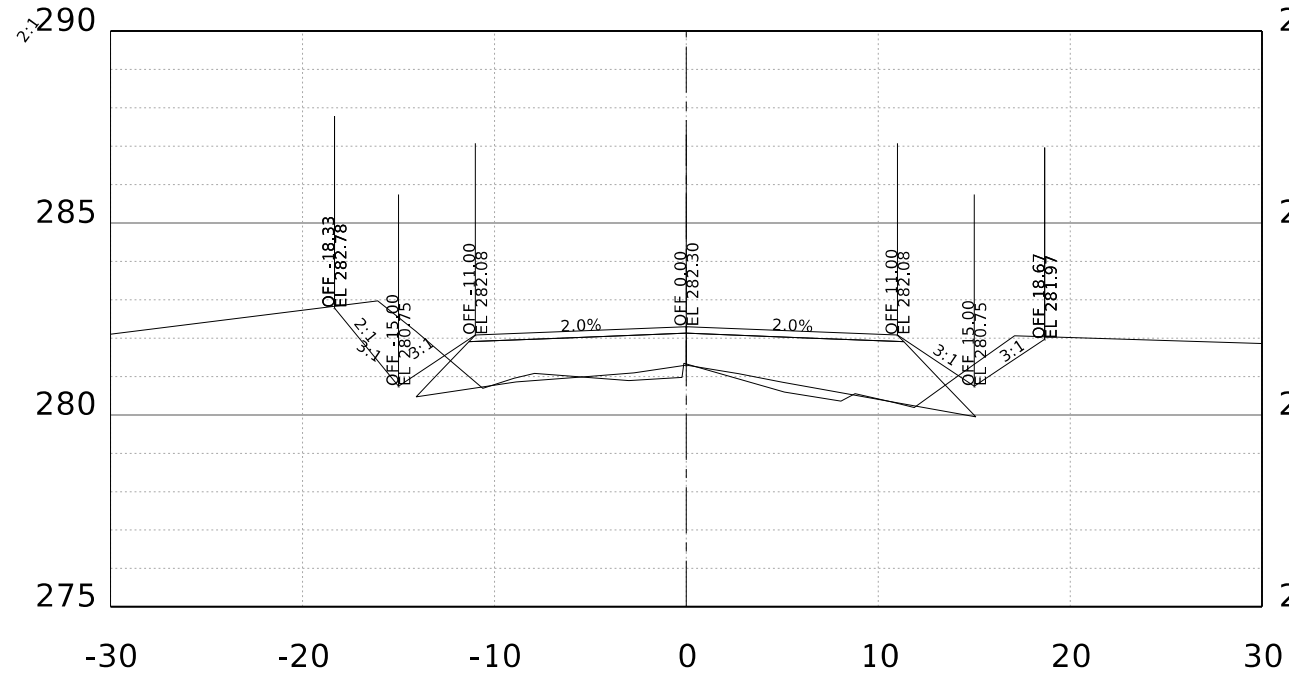
STA. 102+00.00 R1
