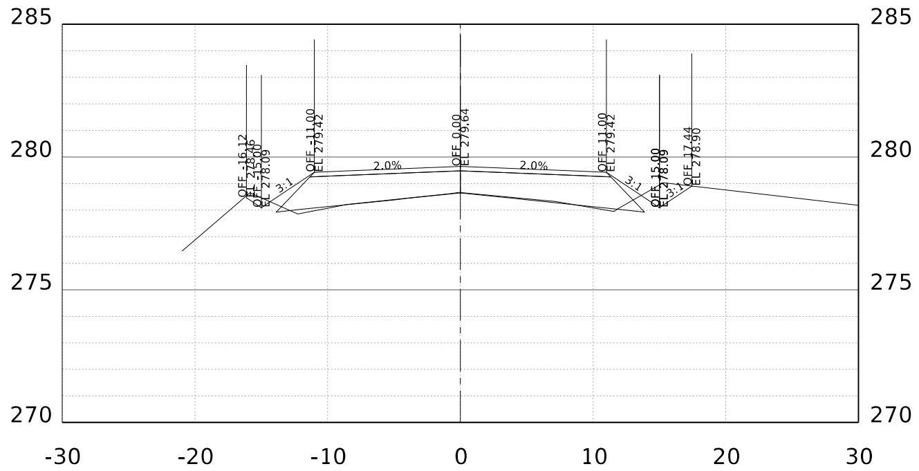
STA. 134+00.00 R1
