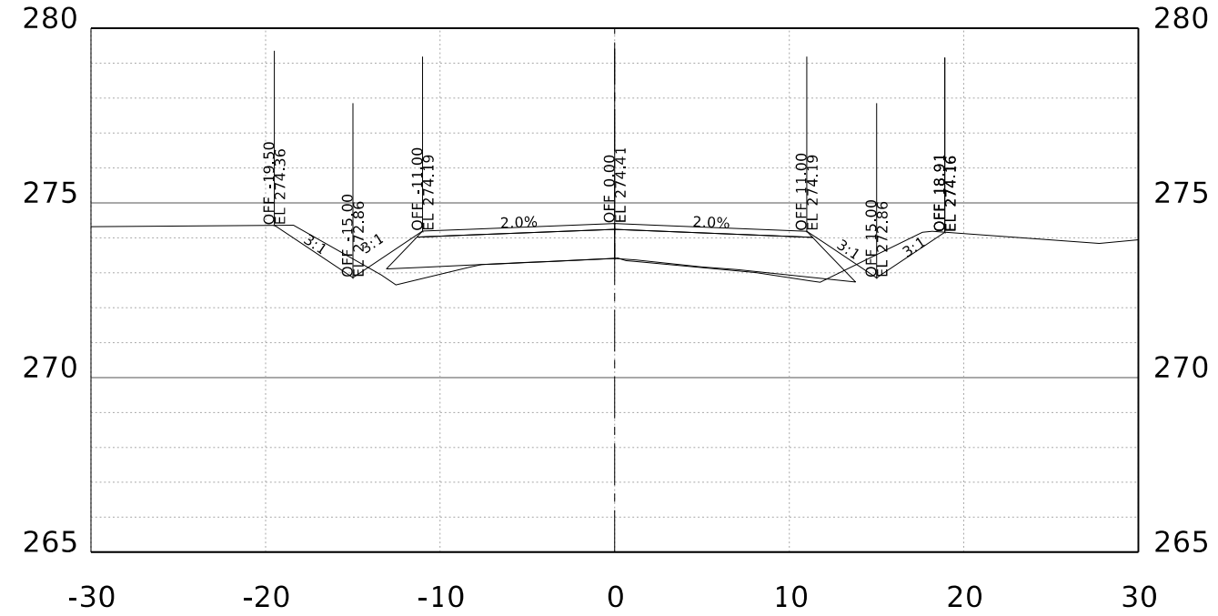
STA. 98+00.00 R1
