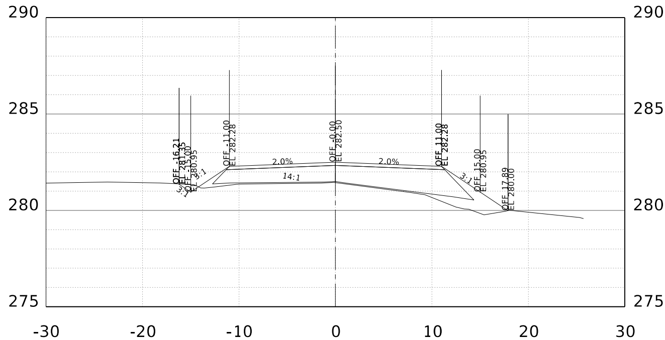
STA. 116+00.00 R1
