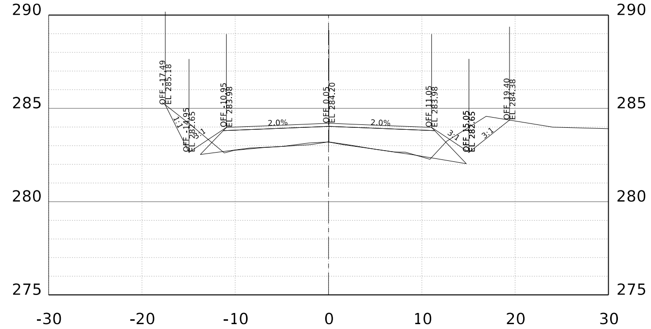
STA. 23+00.00 R1
