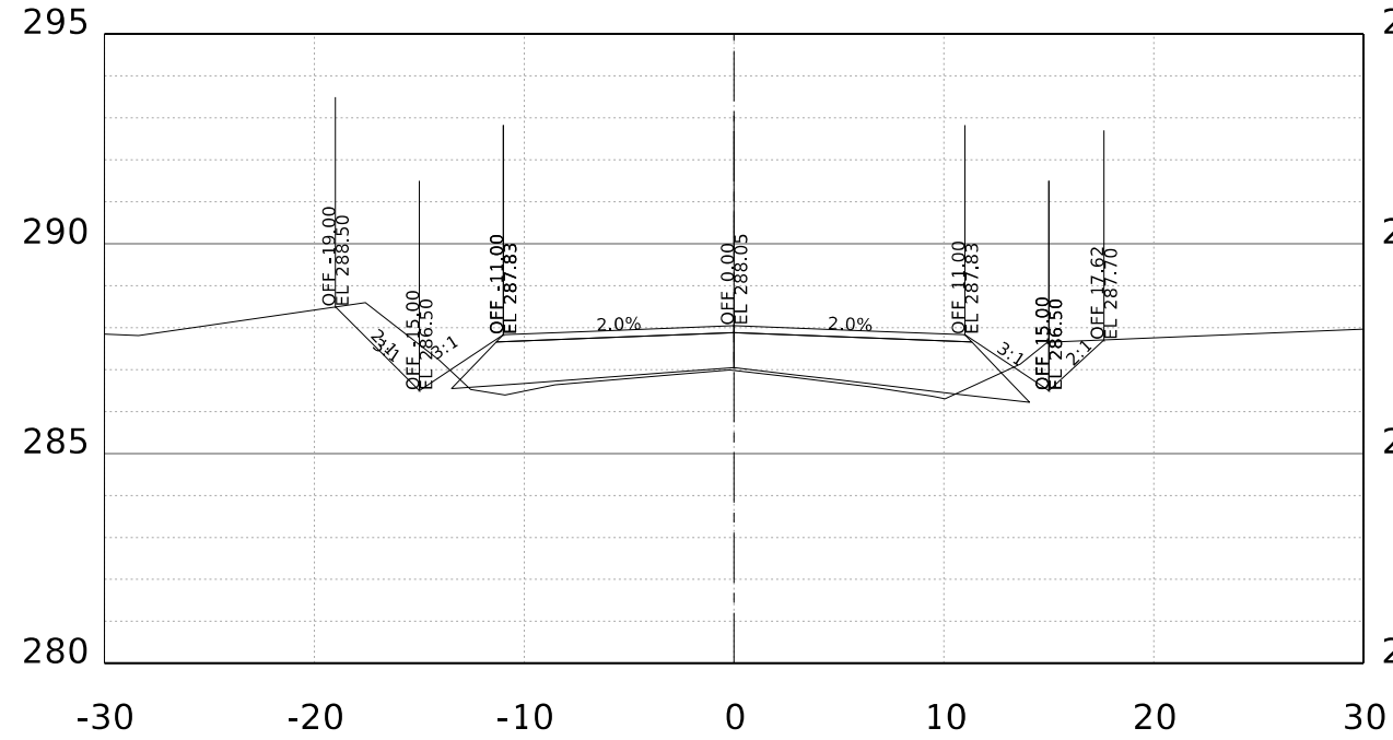
STA. 107+00.00 R1
