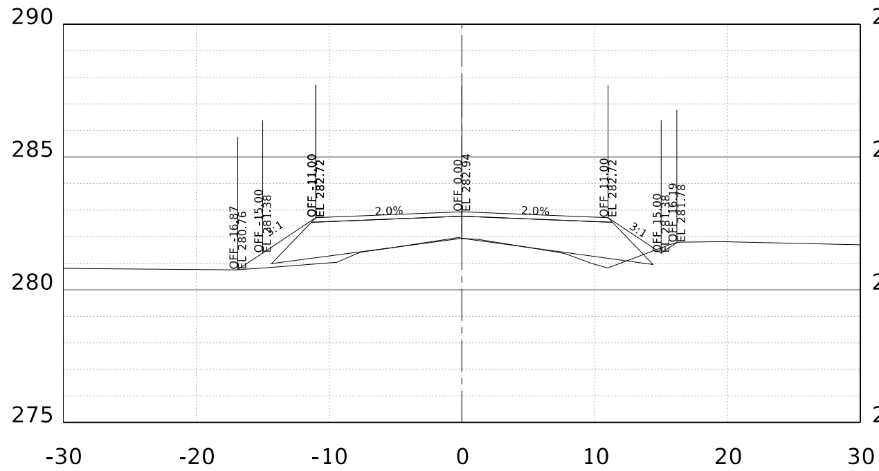
STA. 20+00.00 R1
