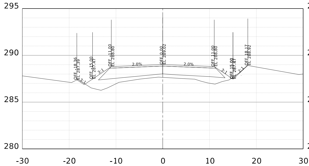
STA. 123+00.00 R1
