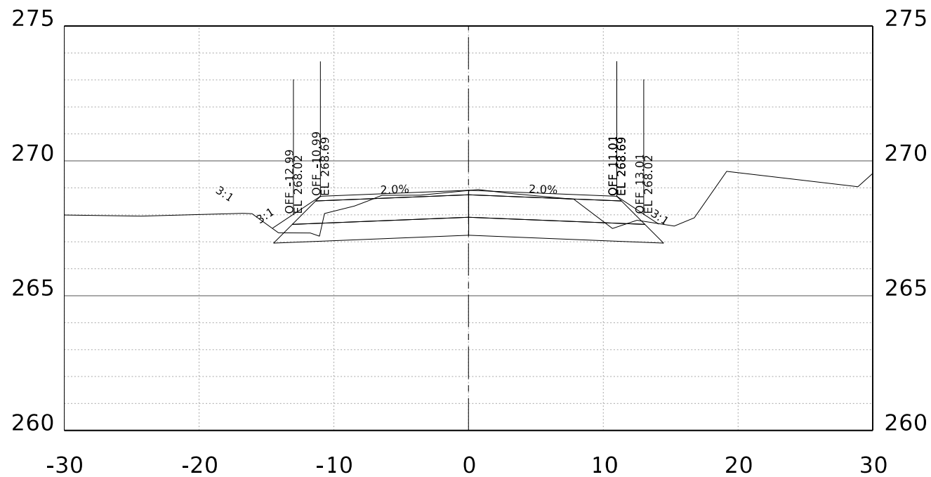
STA. 92+00.00 R1
