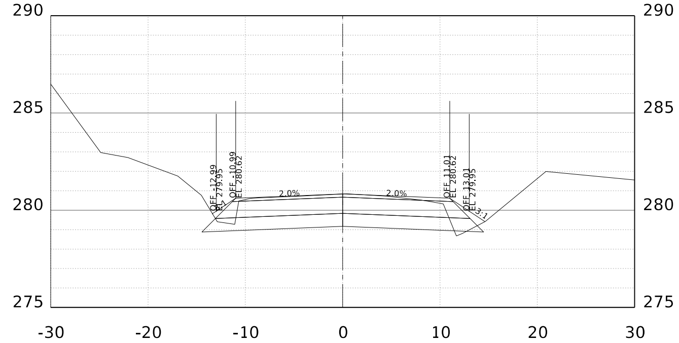
STA. 30+00.00 R1
