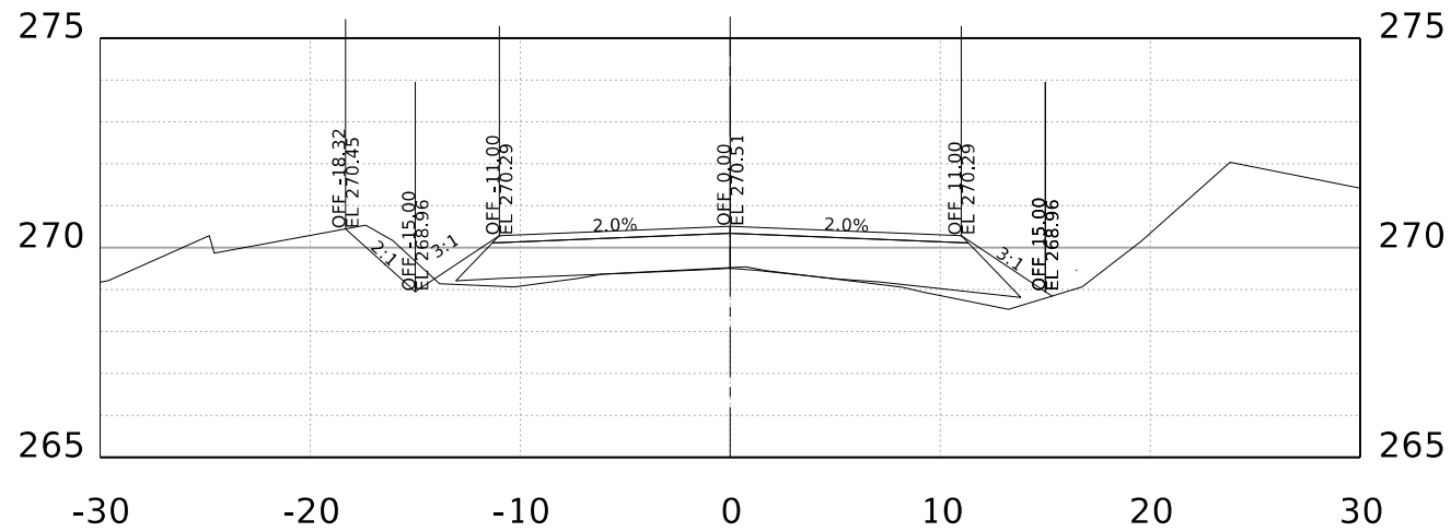
STA. 93+00.00 R1
