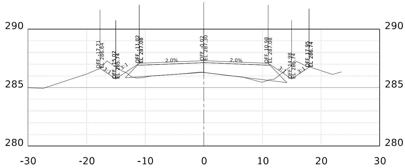
STA. 121+00.00 R1
