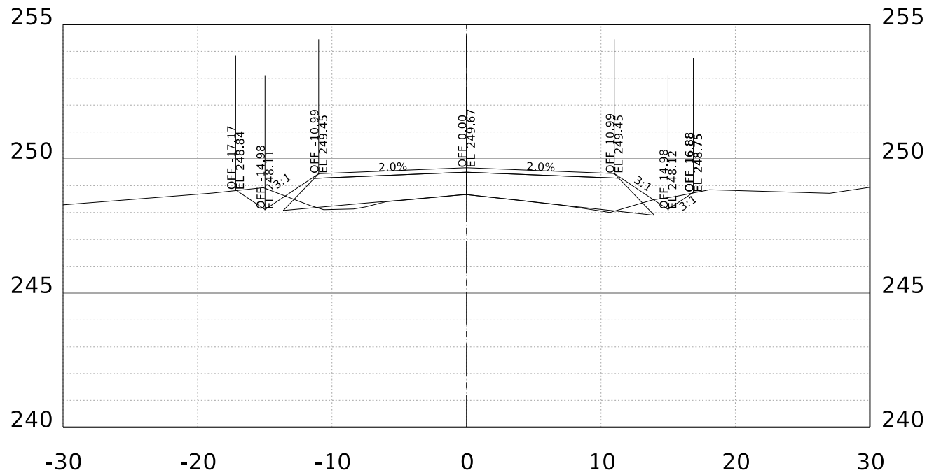
STA. 72+00.00 R1
