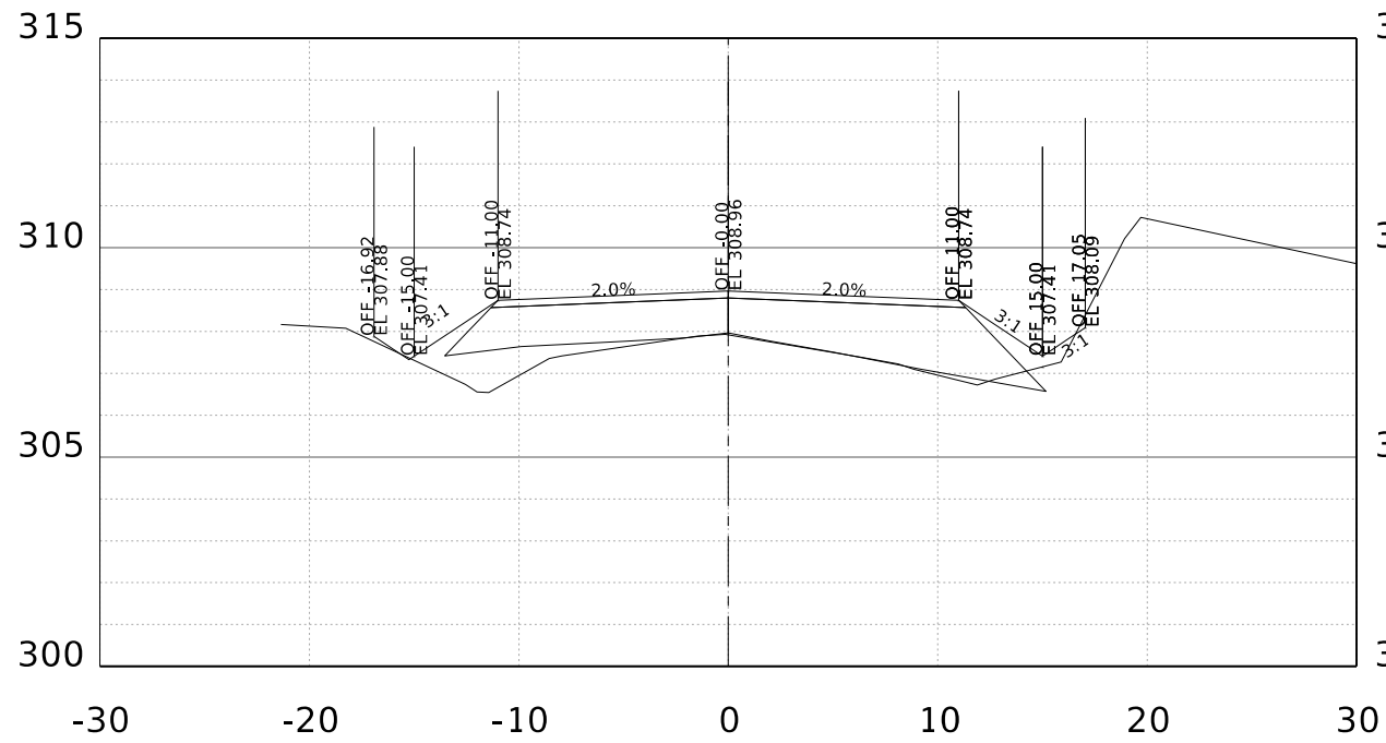
STA. 7+00.00 R1
