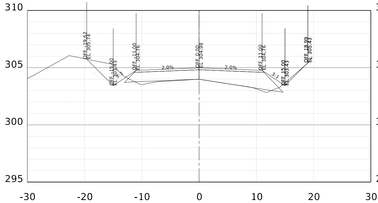
STA. 9+00.00 R1
