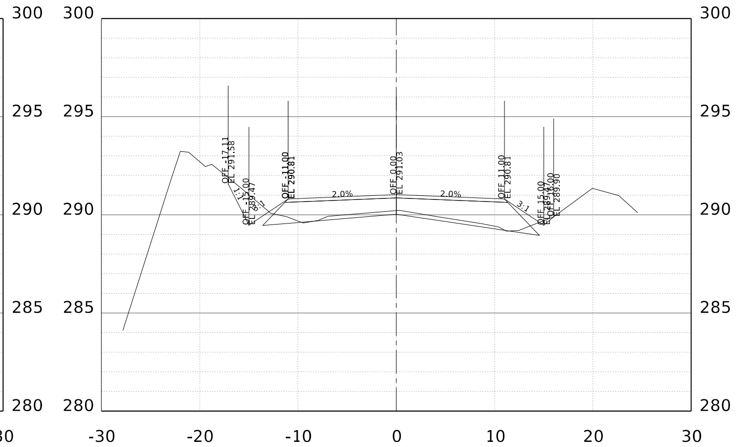
STA. 38+00.00 R1
