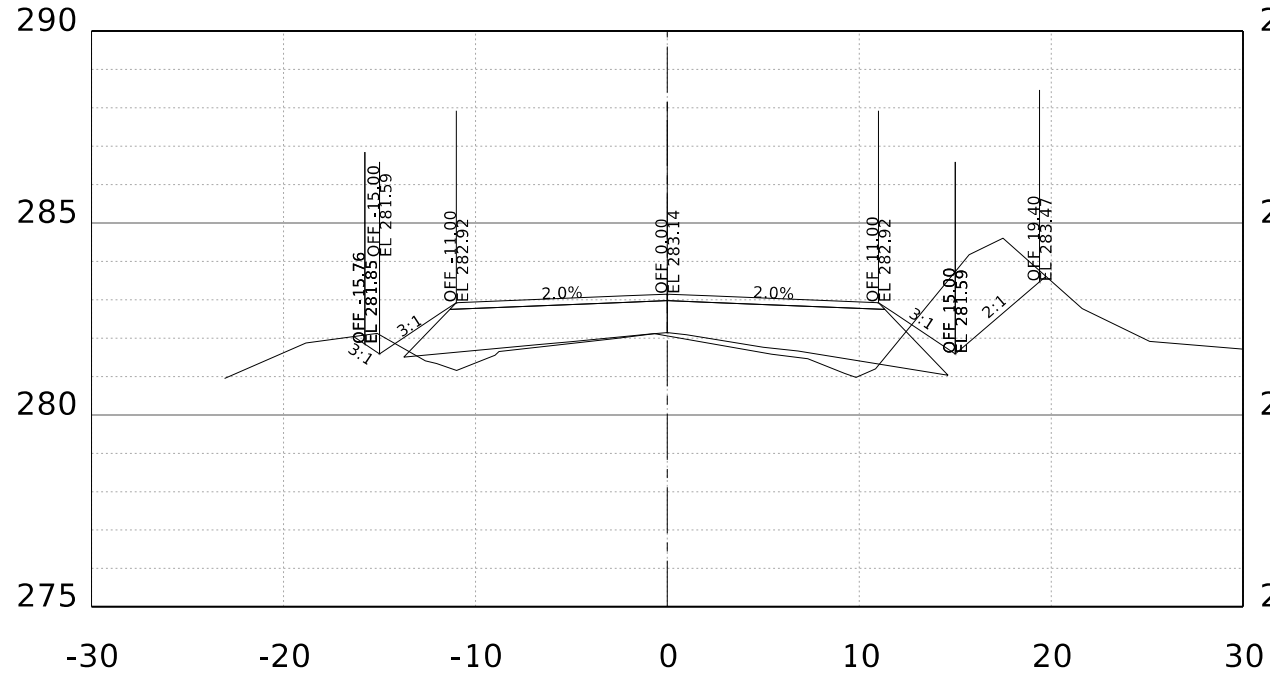
STA. 131+00.00 R1
