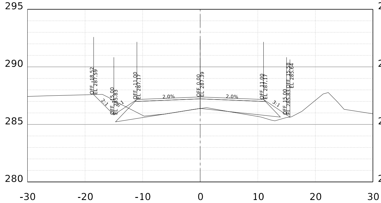
STA. 25+00.00 R1
