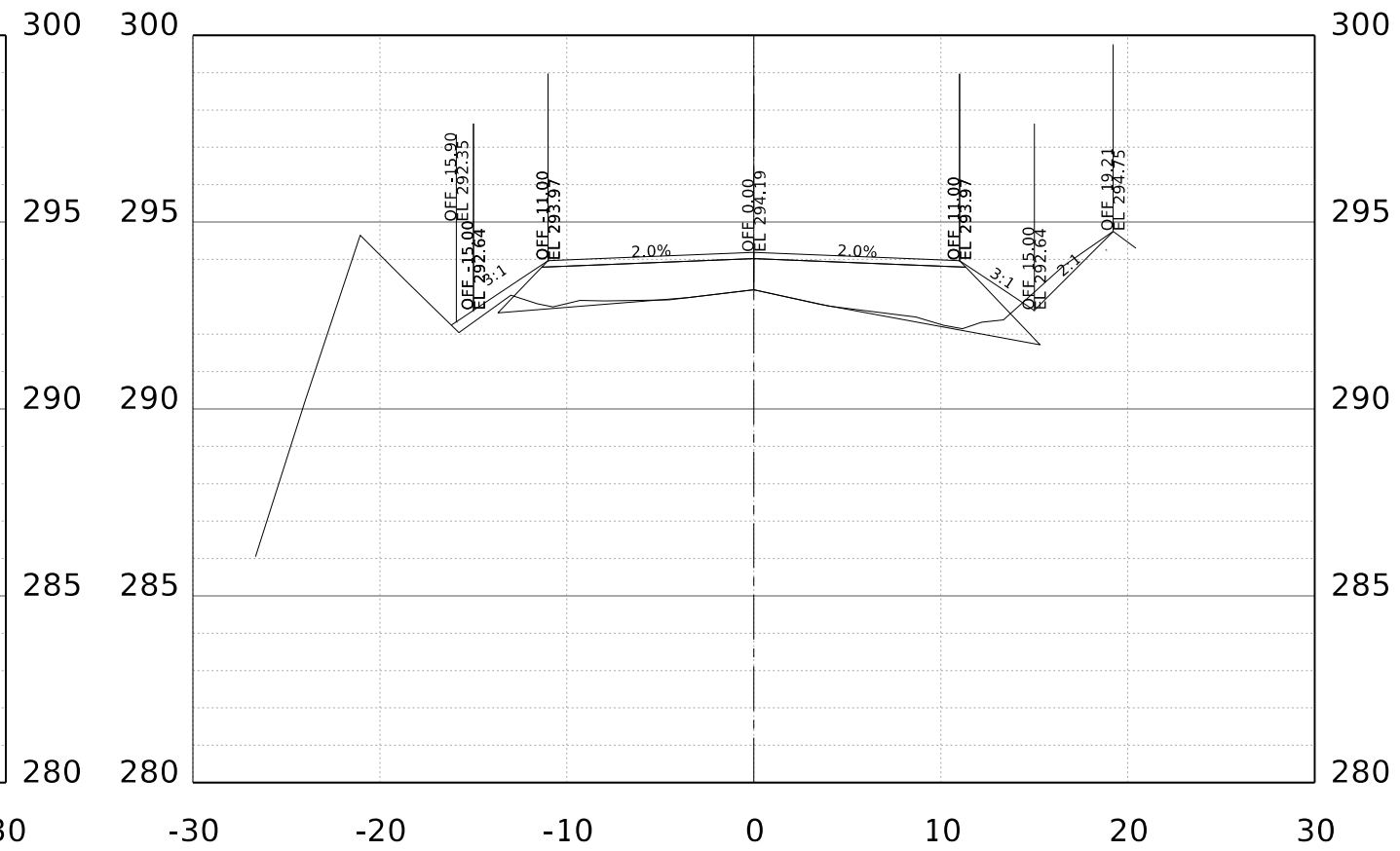
STA. 36+00.00 R1
