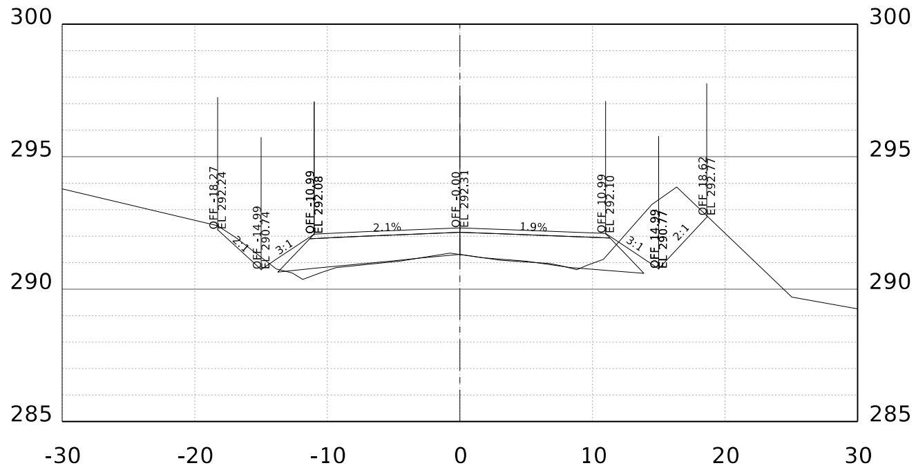
STA. 124+00.00 R1
