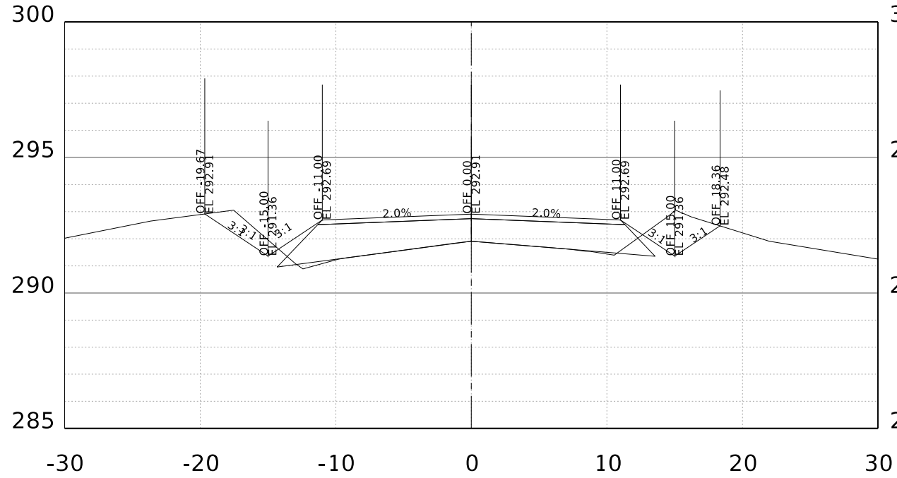
STA. 110+00.00 R1
