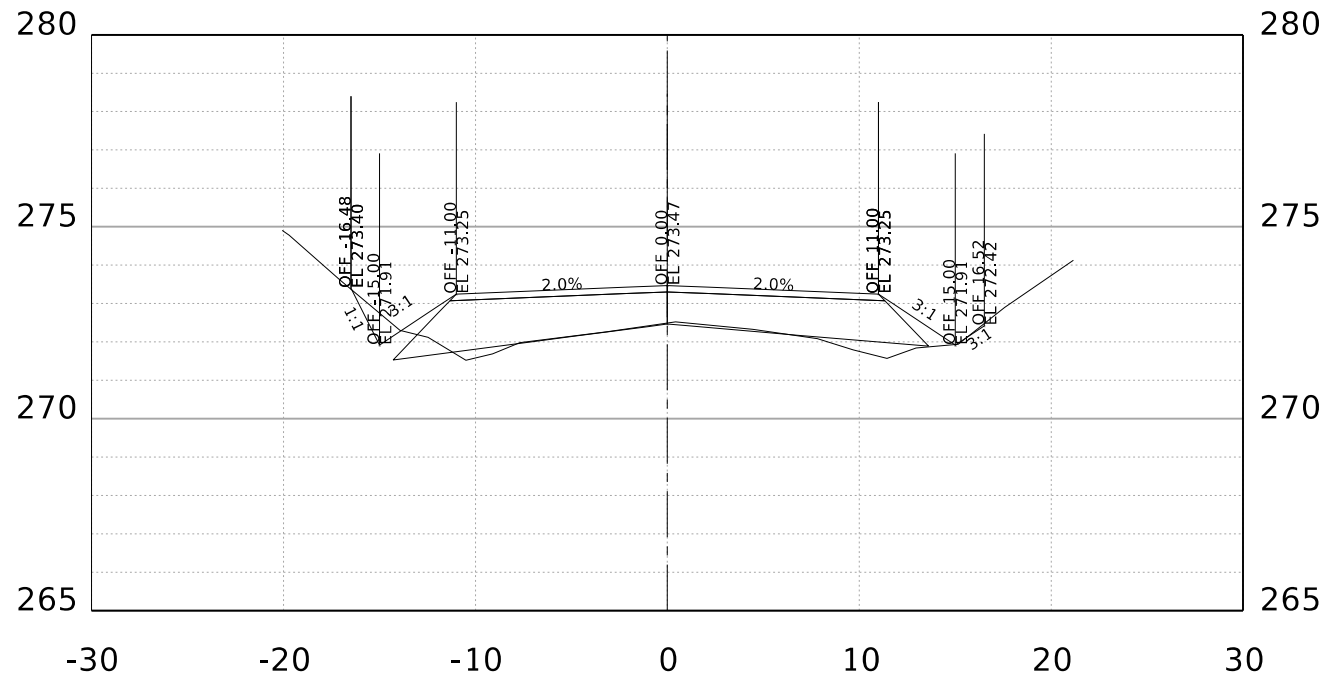
STA. 51+00.00 R1
