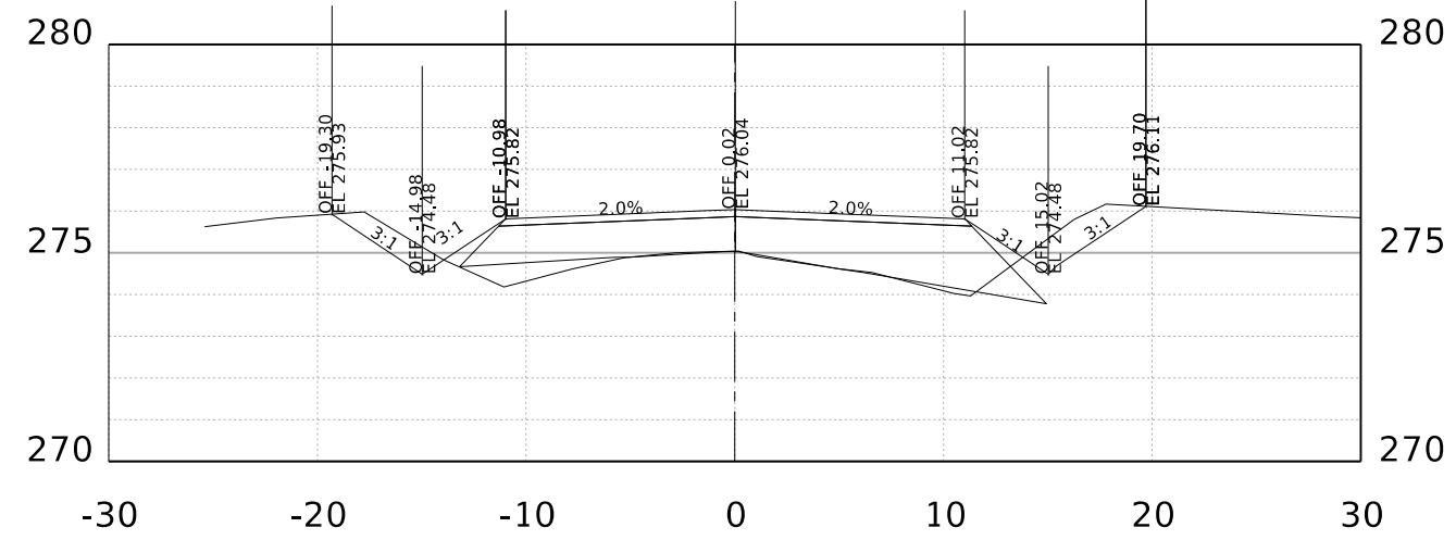
STA. 99+00.00 R1
