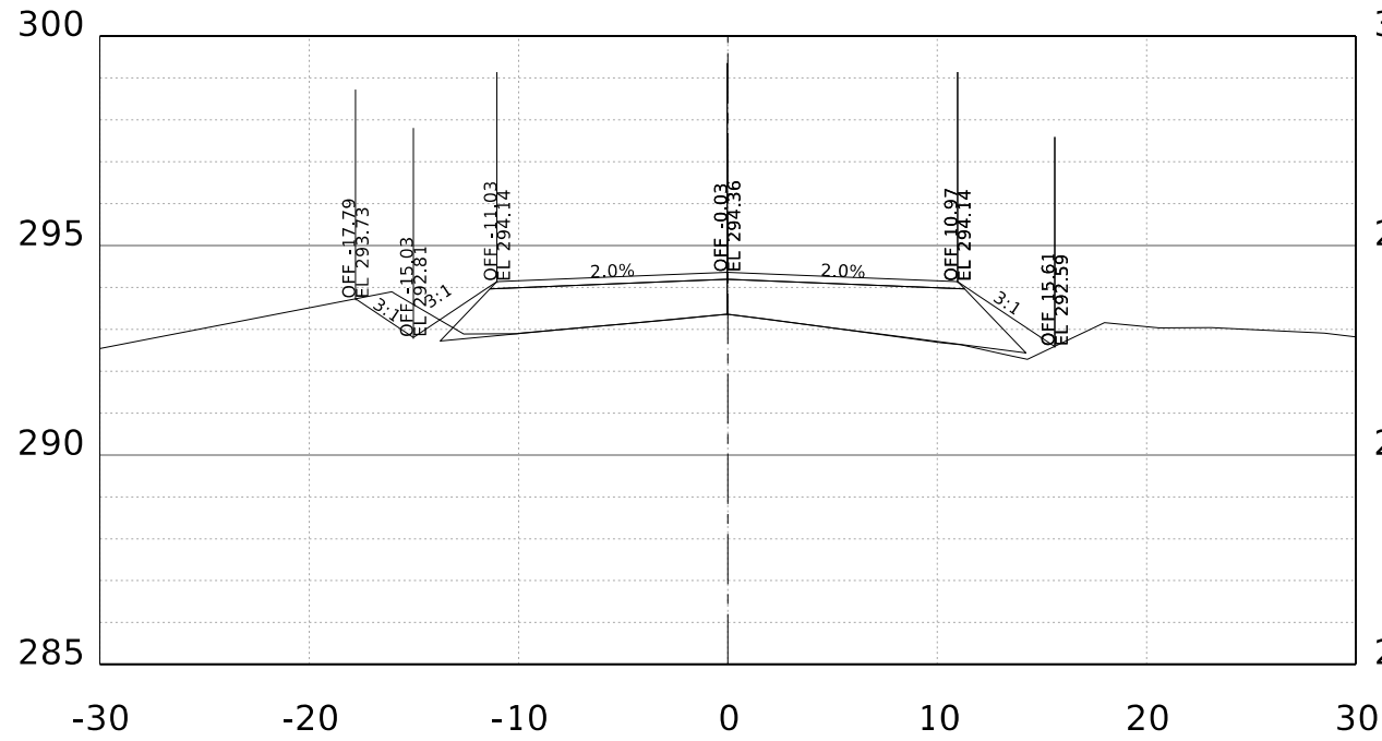
STA. 112+00.00 R1
