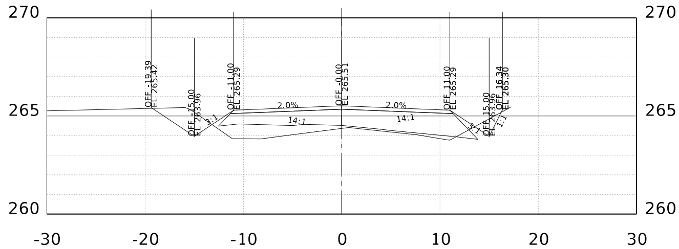
STA. 86+00.00 R1
