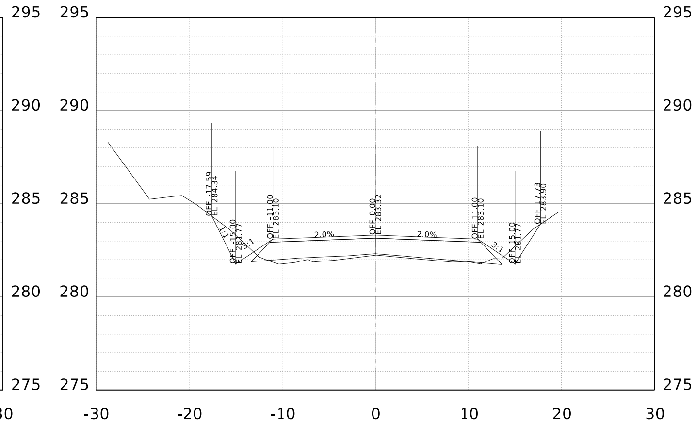
STA. 32+00.00 R1
