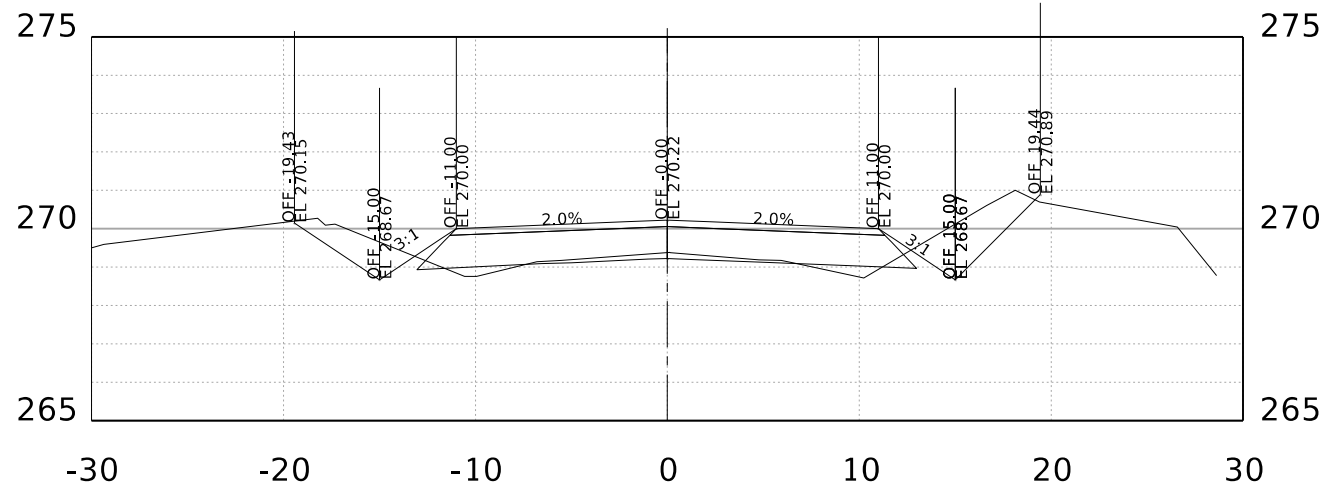
STA. 89+00.00 R1
