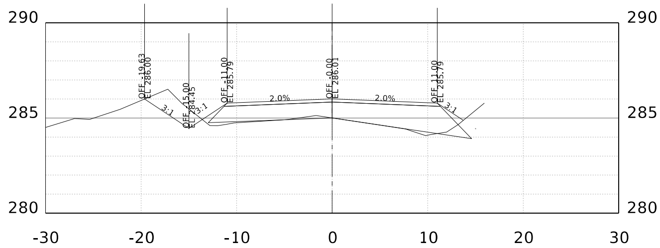
STA. 120+00.00 R1
