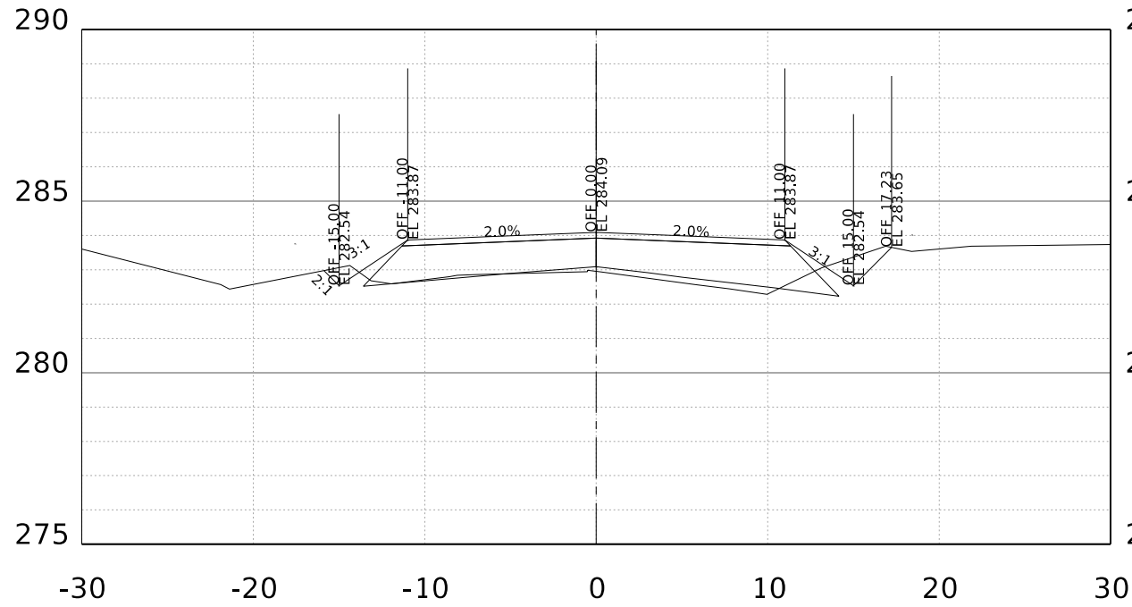
STA. 18+00.00 R1
