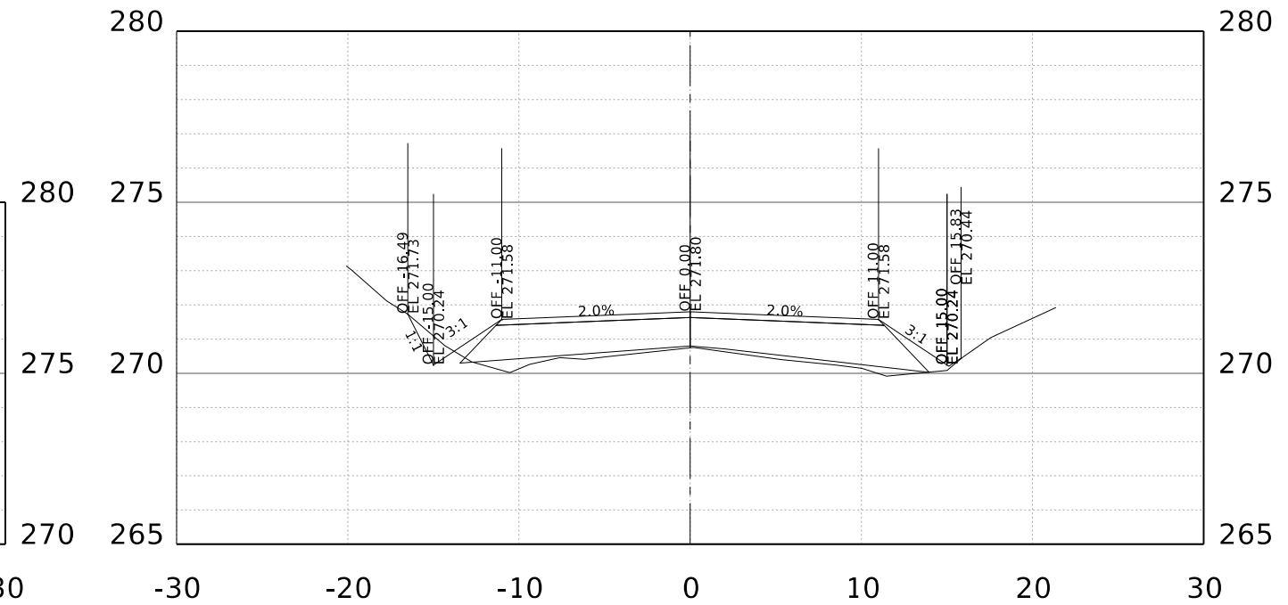
STA. 52+00.00 R1
