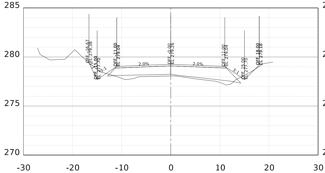
STA. 41+00.00 R1
