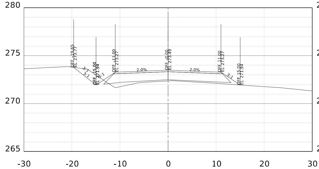
STA. 97+00.00 R1
