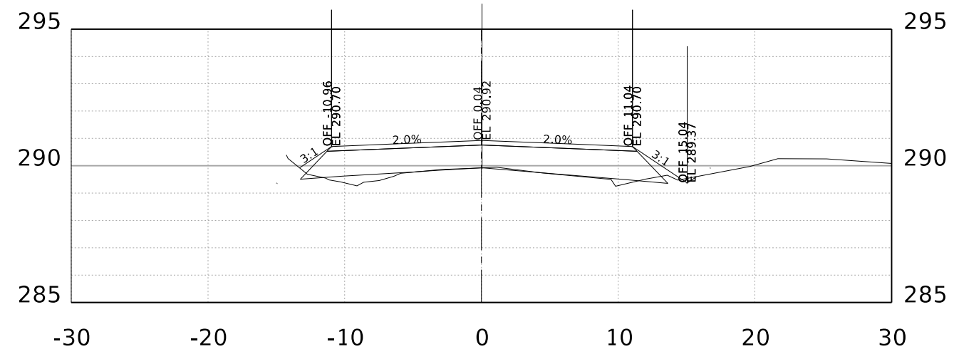
STA. 127+00.00 R1
