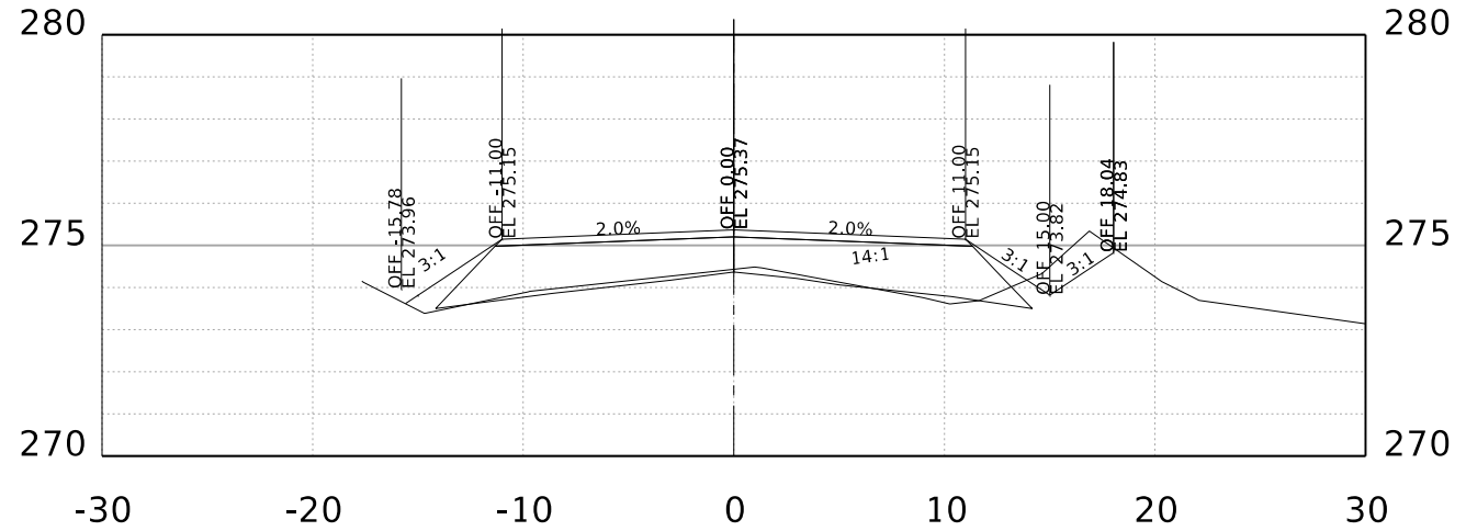
STA. 138+00.00 R1
