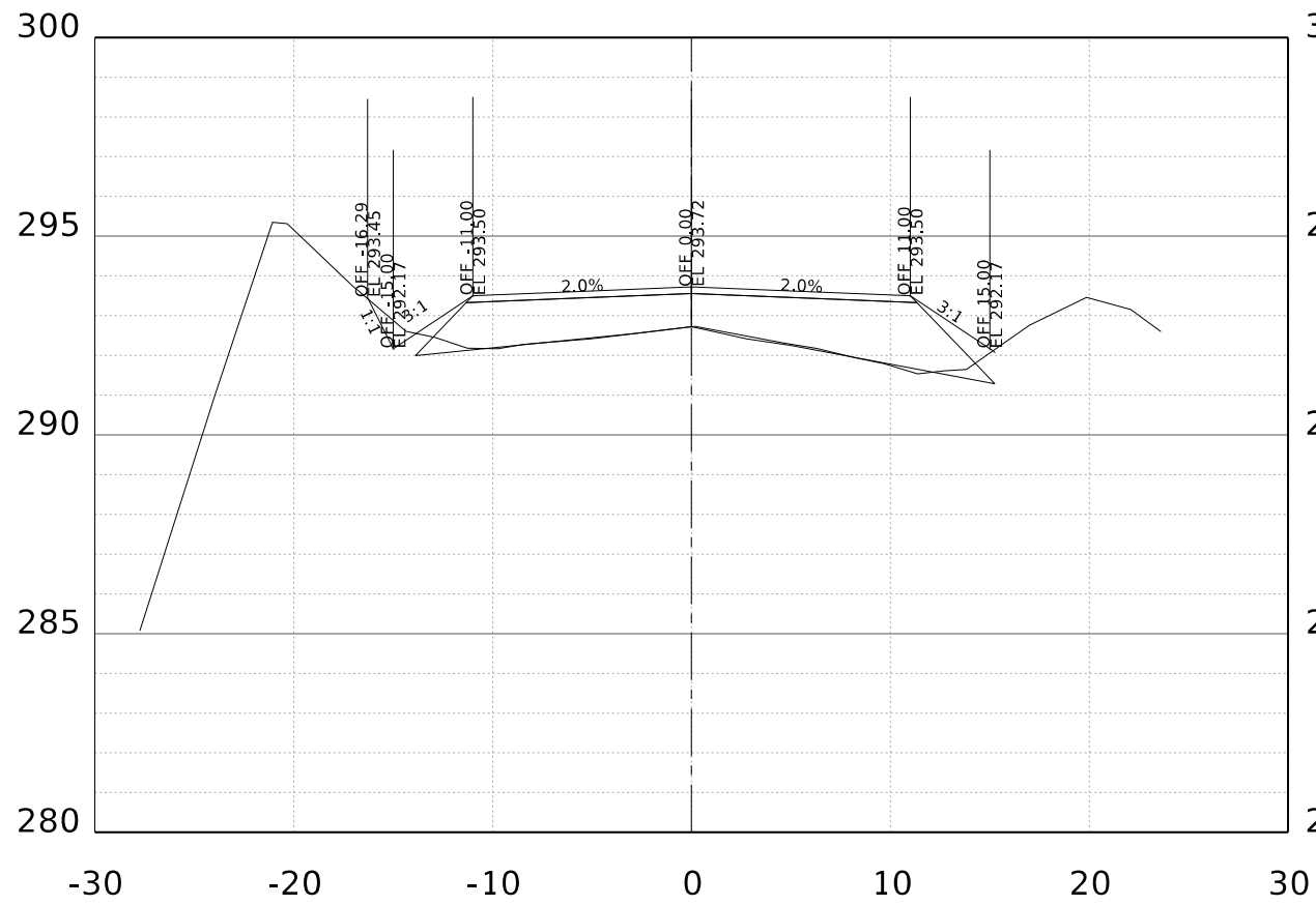
STA. 37+00.00 R1
