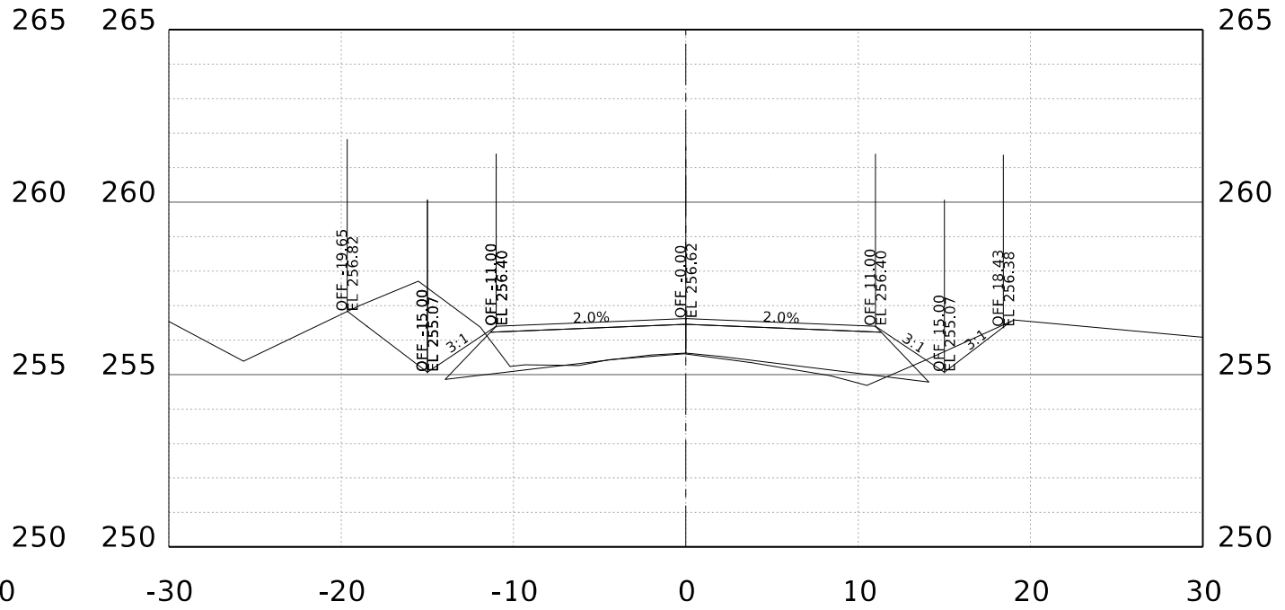
STA. 62+00.00 R1
