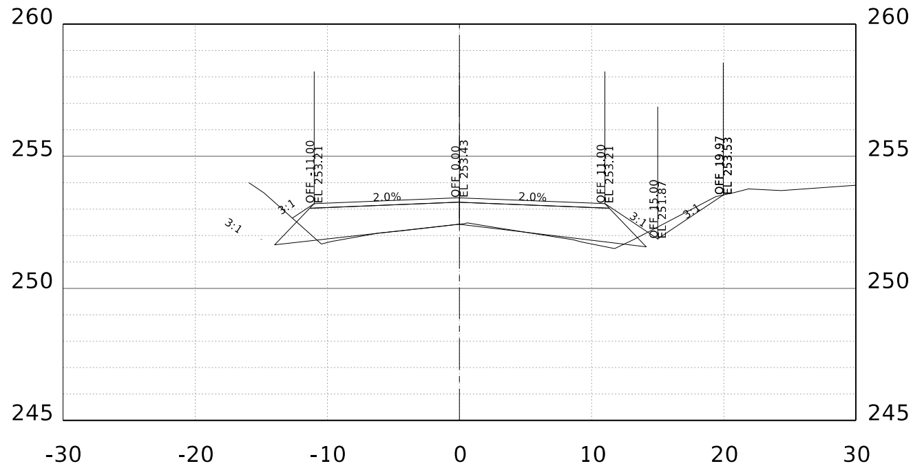
STA. 77+00.00 R1
