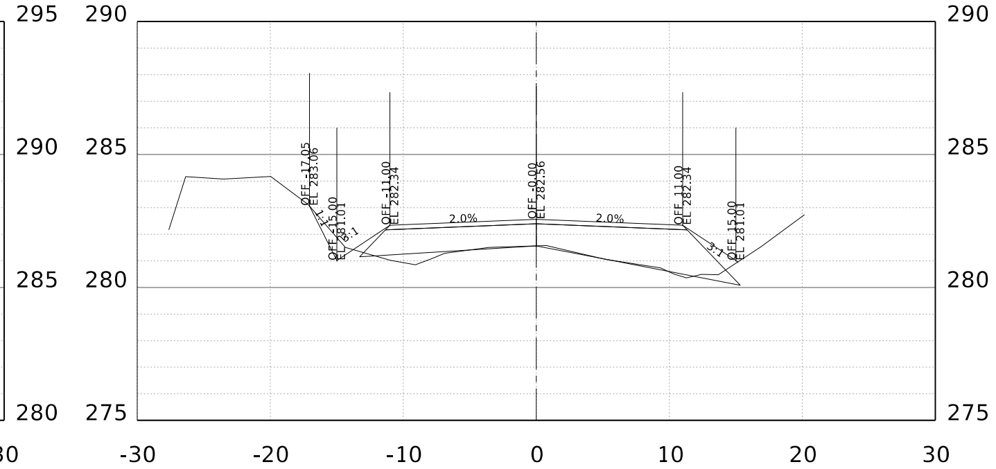
STA. 40+00.00 R1
