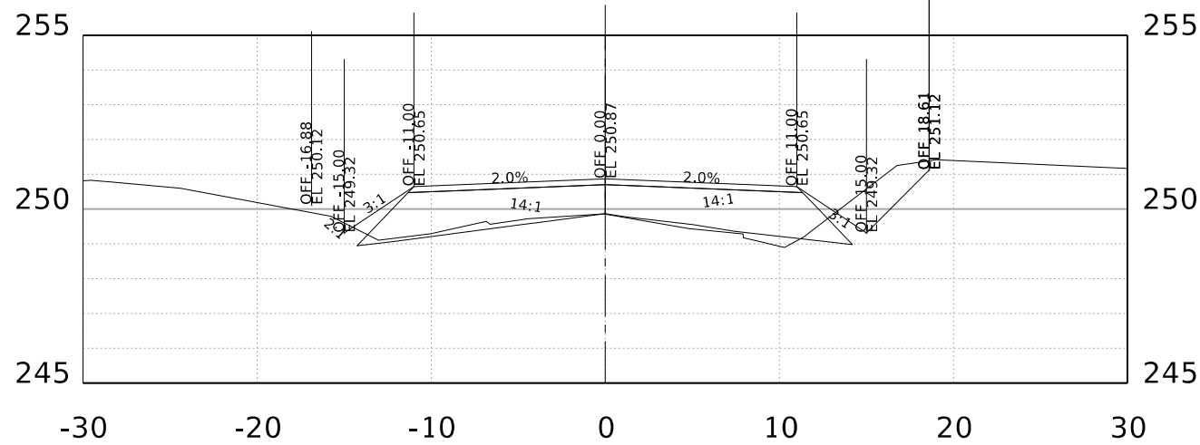
STA. 74+00.00 R1
