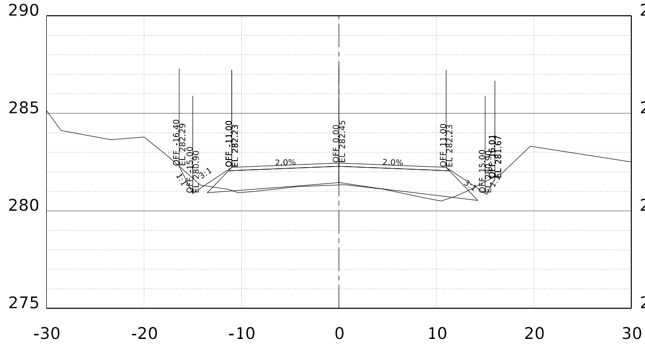
STA. 29+00.00 R1
