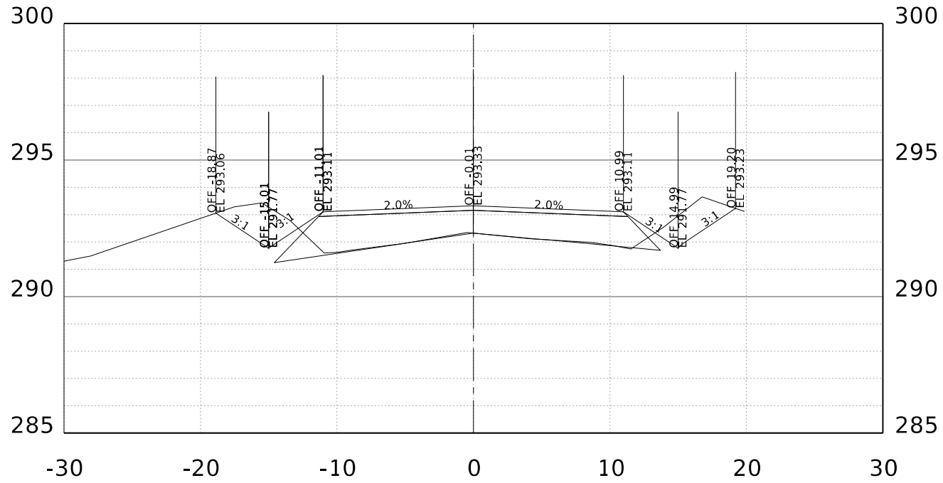
STA. 113+00.00 R1
