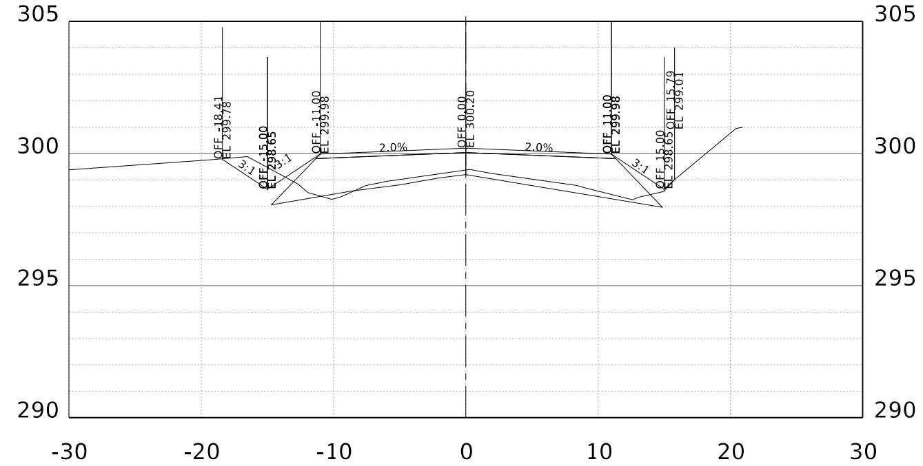
STA. 12+00.00 R1
