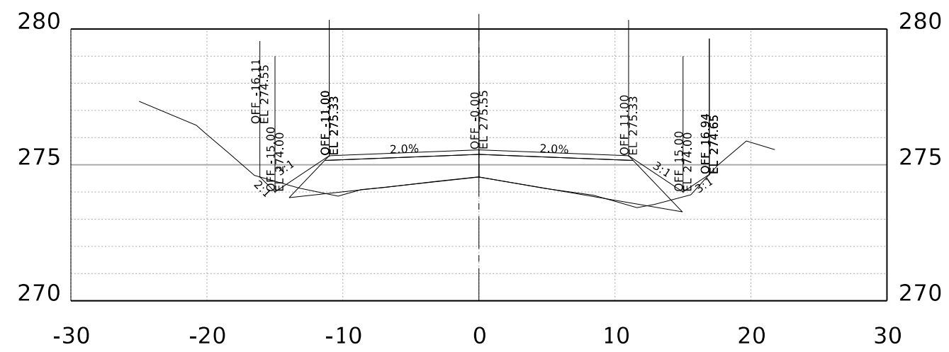
STA. 45+00.00 R1
