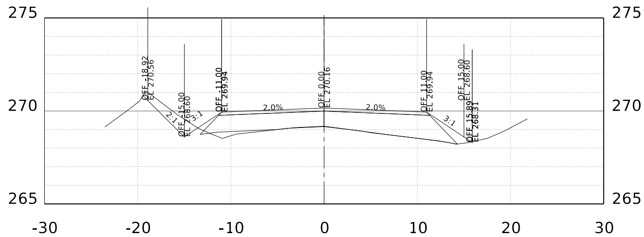
STA. 54+00.00 R1
