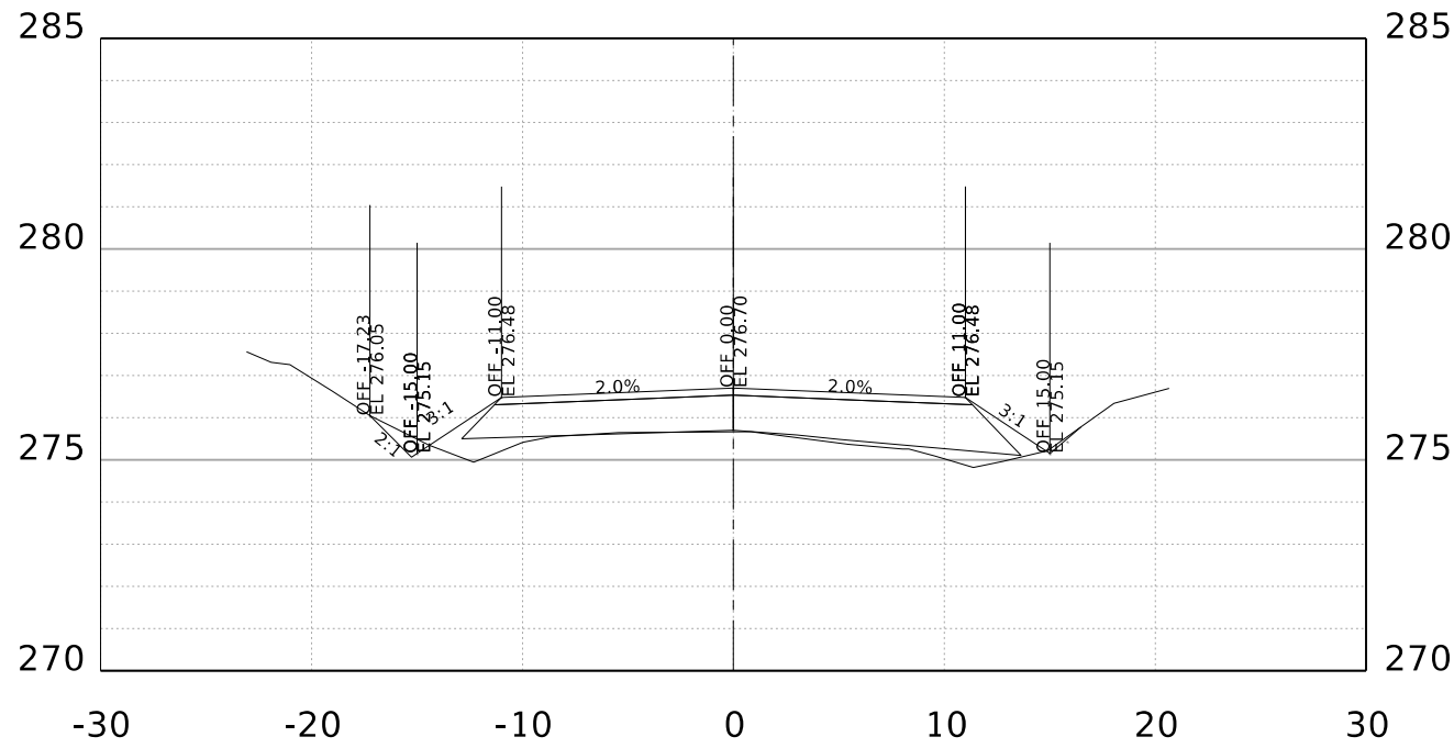
STA. 47+00.00 R1
