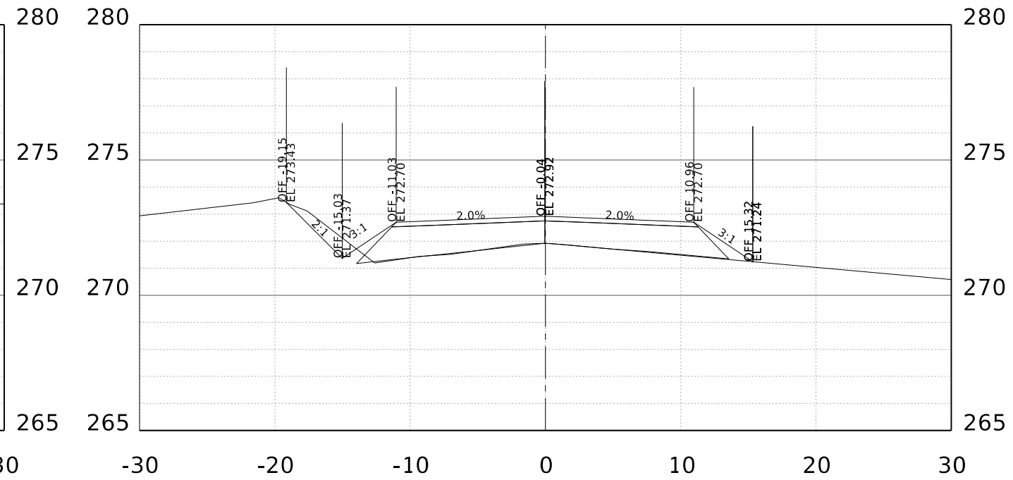
STA. 96+00.00 R1
